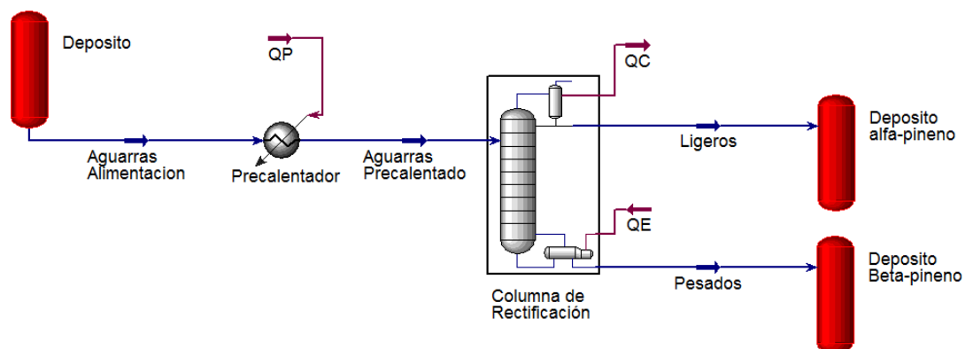
Ilustración 1 Esquema planta de rectificación de aguarrás natural
