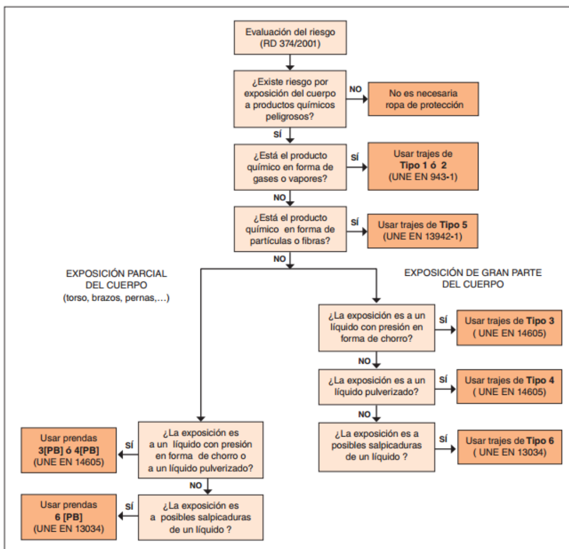
Ilustración 4 Diagrama general del proceso de selección de ropa de protección contra productos químicos NTP 929
