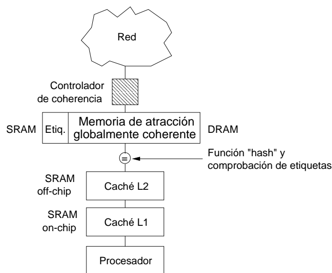
Figura 2.4: Arquitectura de un nodo en un sistema de acceso a memoria sólo cache (COMA).
