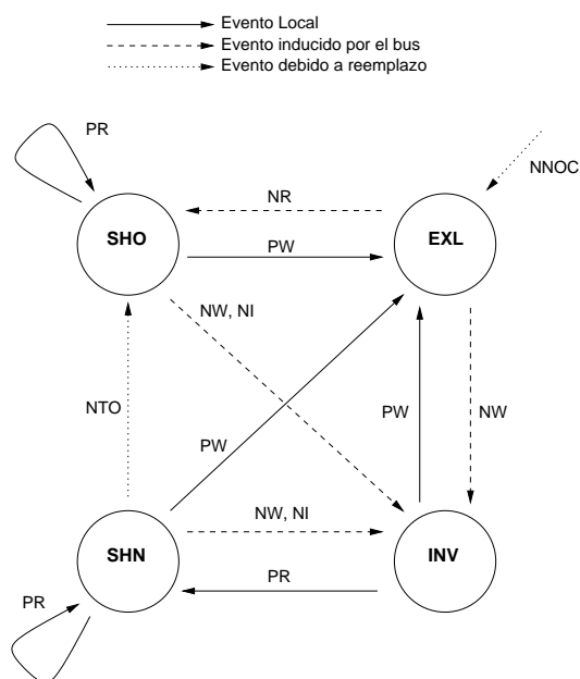
Figura 3.5: Protocolo de coherencia de DICE, según [15].
