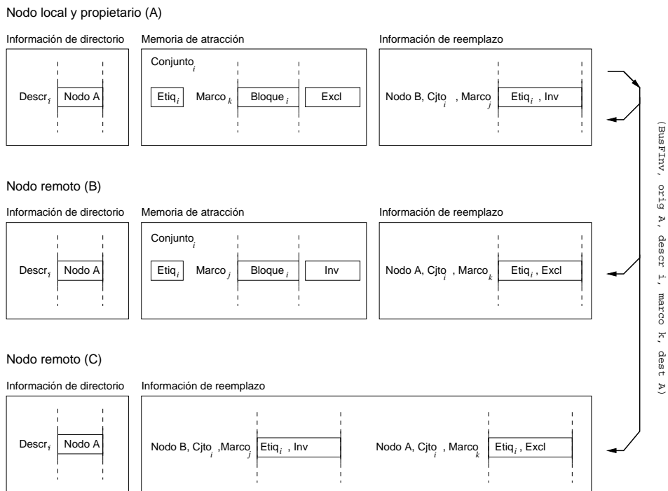
Figura 4.6: Situación final en una solicitud de invalidación rápida. El nodo local y propietario (A) lanza un evento BusFInv. Cuando los nodos remotos lo reciben, actualizan la información de reemplazo correspondiente al nodo local y la correspondiente al resto de nodos que posean una copia. Además, si poseen una copia del bloque, la invalidan. El bloque pasa a Excl en el nodo propietario.
