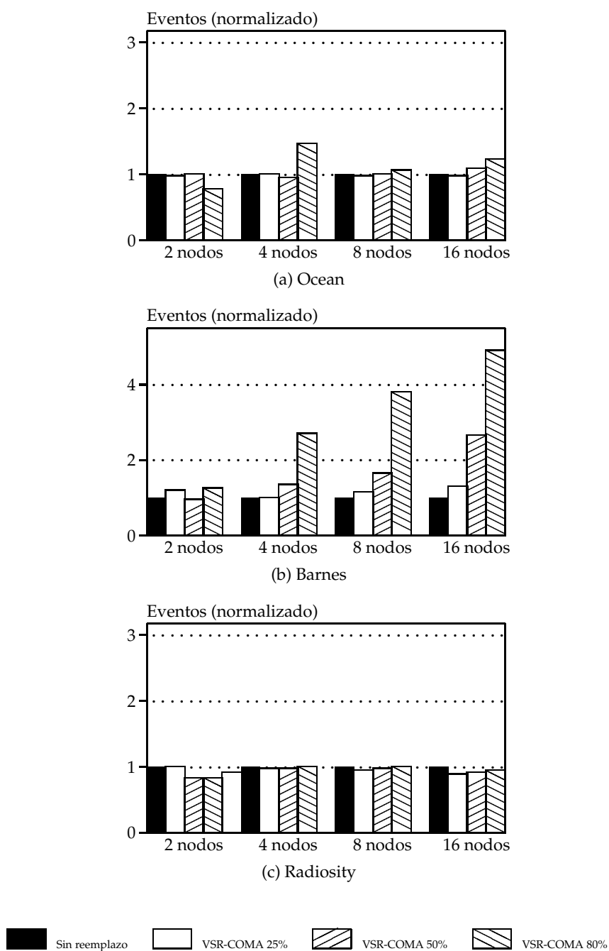
Figura 6.3: Evolución del tráfico para VSR-COMA a diferentes presiones de memoria y con una asociatividad de 8 vías. Los resultados están normalizados respecto a los eventos generados por el sistema sin reemplazo para cada número de nodos.
