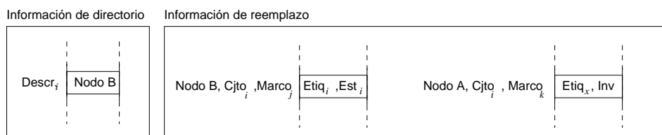
Figura 4.7: Situación inicial en una solicitud de bloque para escritura. El nodo A desea escribir un dato presente en el bloque cuyo descriptor es Descr_i , compuesto por la etiqueta Etiqu_i y el identificador de conjunto Cjto_i . El estado Est_i en el nodo propietario B será igual a Excl o SharOwn. El resto de nodos del sistema se comportan como nodos remotos.
