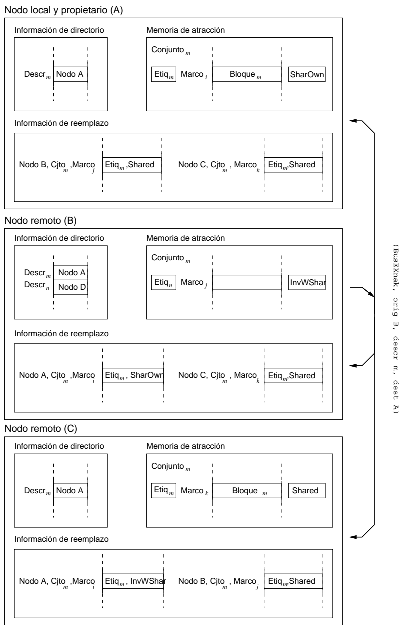
Figura 4.14: Recepción de una respuesta negativa de reemplazo (evento BusEXnak). El nodo propietario del bloque modifica su estado a SharOwn, y el resto de nodos actualizan la información de reemplazo correspondiente a él.
