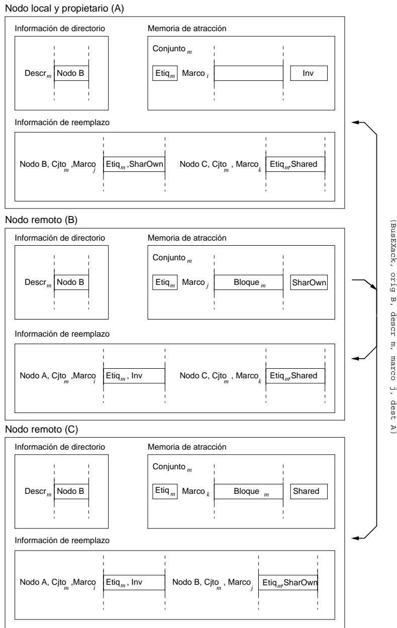
Figura 4.12: Recepción de una respuesta de reemplazo (evento BusEXack). El nodo A y el nodo C actualizan la información de propietario del bloque, junto con la información de reemplazo correspondiente al nodo B. El nodo C, además, actualiza la información de reemplazo del antiguo y del nuevo propietario. El nodo A invalida el bloque. Ya existe un marco de bloque Inv en su memoria de atracción, por lo que puede realizarse la operación de memoria pendiente.
