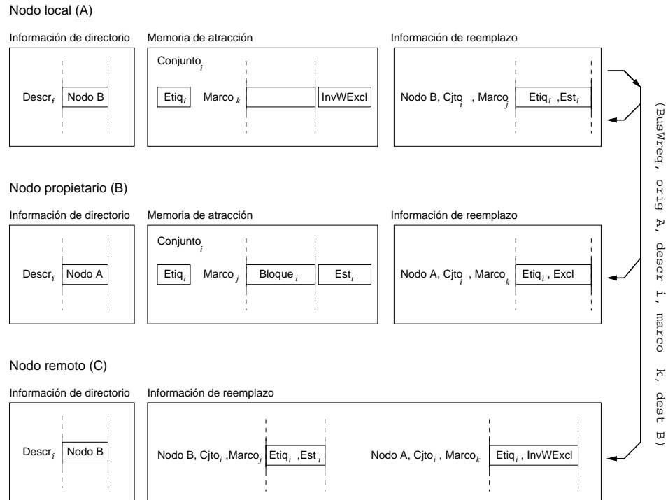
Figura 4.8: Recepción de una solicitud de bloque para escritura (evento BusWReq). Cuando el nodo local (A) envía la solicitud, se actualiza la información de reemplazo correspondiente al nodo local en todos los nodos remotos (pasa a InvWExcl, a la espera de que se confirme la respuesta del propietario del bloque). En el nodo propietario (B) se modifica la información de reemplazo de modo que el estado de Marco k en el nodo A pase a Excl. También se modifica la información de directorio en el nodo B, pasando a ser el nodo local (A) el nuevo propietario. El bloque se invalidará en el nodo B en cuanto dicho nodo envíe la respuesta BusWack.
