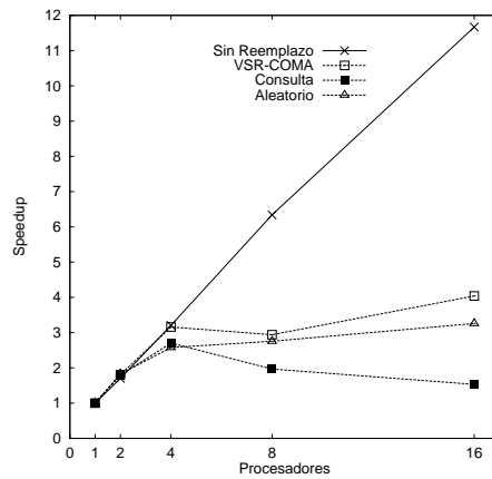
(d) Barnes
