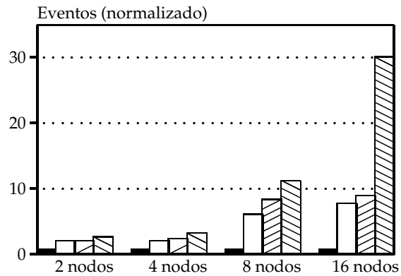
(b) LU
