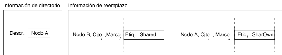
Figura 4.5: Situación inicial en una solicitud de invalidación rápida. El nodo local y propietario (A) posee una copia del bloque en SharOwn, lo que indica que puede haber otras copias válidas del bloque en el sistema. El nodo remoto B posee una de esas copias, mientras que el nodo remoto C no posee ninguna.
