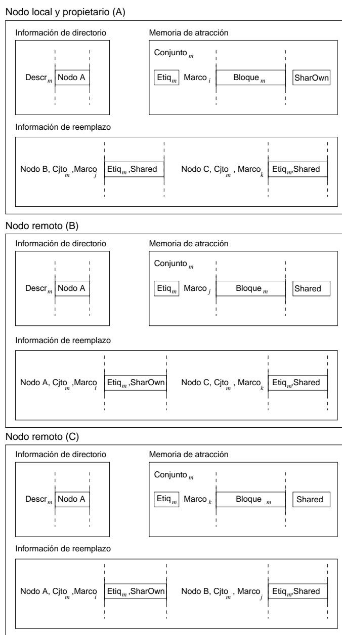
Figura 4.10: Situación previa al desalojo de un bloque. El nodo A desea desalojar el bloque cuyo descriptor es Descr m y que se encuentra en estado SharOwn. Tiene dos posibilidades: enviarlo al nodo B o al nodo C. Ambos poseen una copia Shared del bloque, por lo que ambas opciones son equivalentes. La selección del nodo destino dependerá del algoritmo de selección correspondiente.
