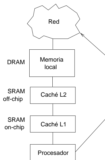
Figura 2.2: Arquitectura de un nodo en un sistema de memoria virtual compartida distribuida (DVSM).
