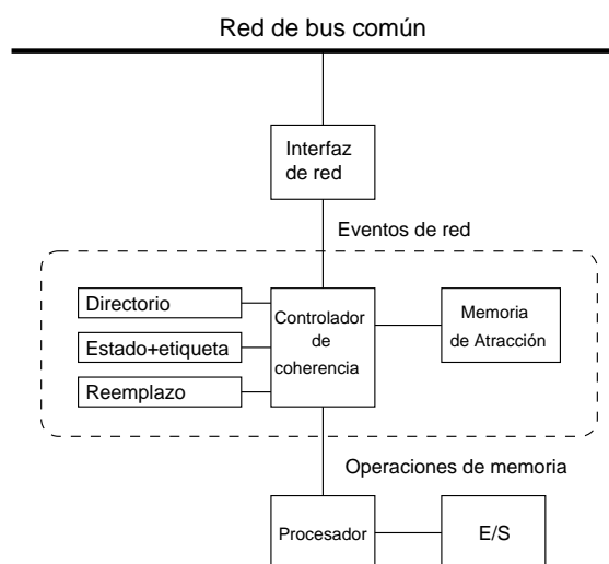
Figura 4.1: Estructura de un nodo de proceso en VSR-COMA.
