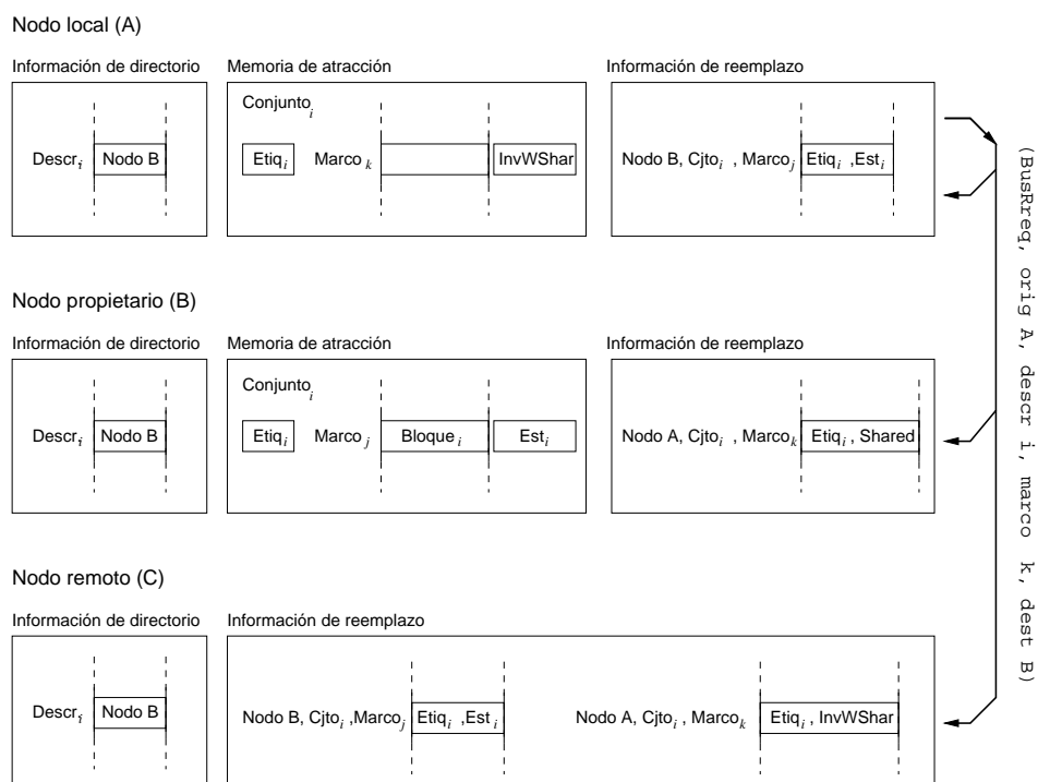
Figura 4.3: Recepción de una solicitud de lectura (evento BusRreq). Cuando el nodo local A envía la solicitud al nodo B, se actualiza la información de reemplazo correspondiente al nodo local en todos los nodos remotos (pasa a InvWShar, a la espera de que se confirme la respuesta del propietario del bloque). En el nodo propietario B, se modifica la información de reemplazo de modo que el estado del marco k en el conjunto i del nodo A pase a Shared. Cuando el nodo propietario responda enviando el bloque i , deberá cambiar el estado de su copia ( Est_i ) a SharOwn.
