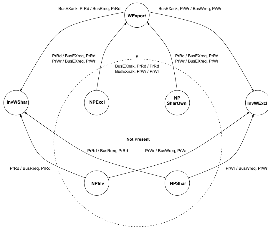
Figura 4.16: Detalle del diagrama de estados de la figura 4.15, para el caso de que el bloque no esté presente en la memoria de atracción.
