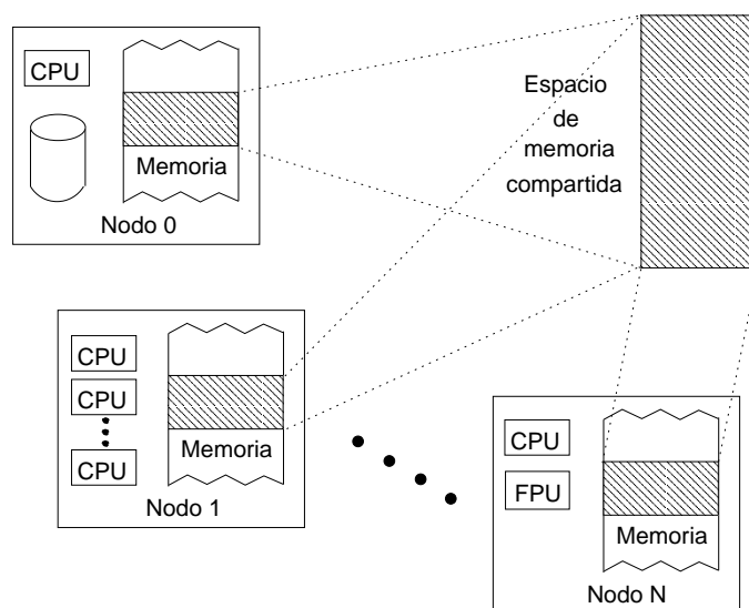
Figura 2.1: Memoria compartida distribuida.
