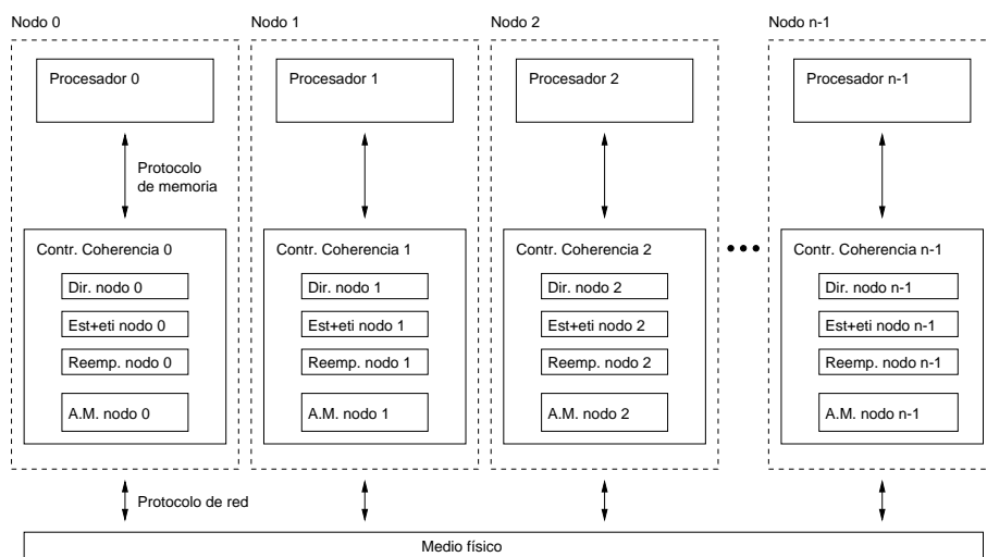
Figura 5.2: Diagrama de bloques del sistema a simular por EMUCOMA.
