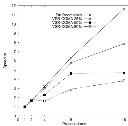
(d) Barnes
