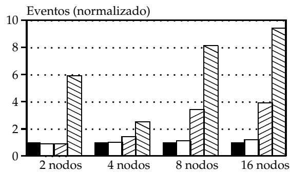
(b) LU
