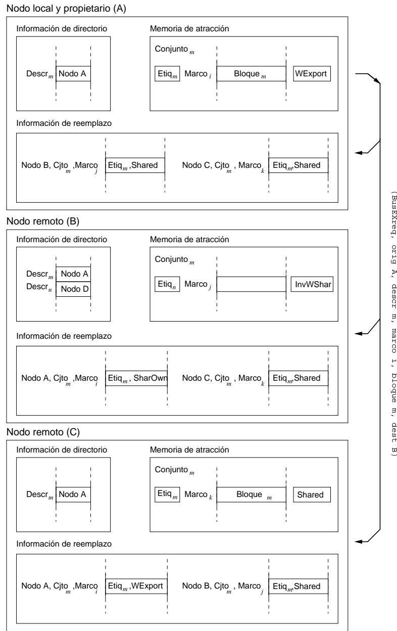
Figura 4.13: Condición de carrera en una solicitud de reemplazo. El estado inicial es el que se muestra en la figura 4.10. Un instante antes de recibir la solicitud de reemplazo del nodo A, el nodo B ha decidido utilizar el marco que ocupa su copia Shared del bloque m para almacenar una copia del bloque n , que será solicitado de forma remota. En consecuencia, cambia el estado del marco j a InvWShar. Cuando llegue la solicitud de desalojo, el nodo B deberá responder negativamente (figura 4.14).
