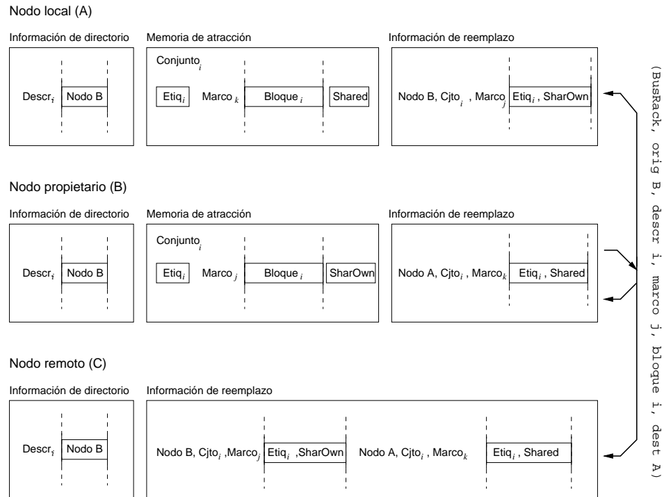
Figura 4.4: Recepción de una respuesta de lectura (evento BusRack). El nodo propietario (B) cambia el estado de su bloque a SharOwn, ya que existe otra copia en el sistema, y envía la respuesta BusRack. Al recibirla, el nodo local copia el bloque en el marco k y coloca el estado en Shared. En todos los nodos remotos se actualiza la información de reemplazo correspondientes al nodo local y al nodo propietario. En el nodo local se actualiza la información de reemplazo del nodo propietario. El estado final tras la operación es el que se muestra en la figura.
