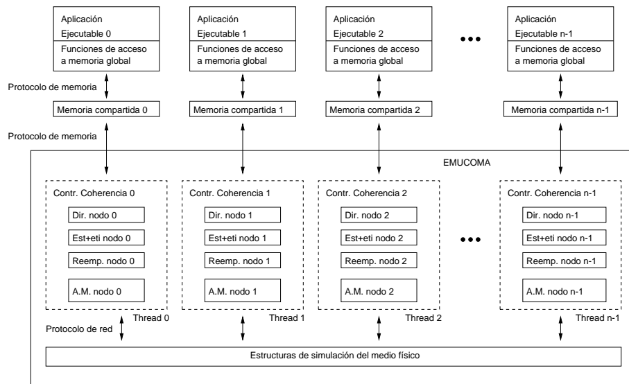
Figura 5.3: Estructura de procesos del simulador EMUCOMA.
