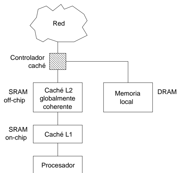
Figura 2.3: Arquitectura de un nodo en un sistema de memoria de acceso no uniforme con caches coherentes (CC-NUMA).
