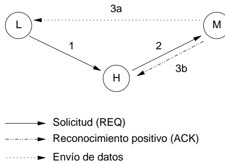
Figura 3.1: Solicitudes de lectura en COMA-F, según [45].
