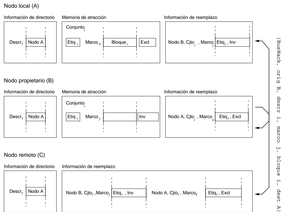
Figura 4.9: Recepción de una respuesta de escritura (evento BusWack). Cuando los nodos reciben este evento actualizan la información de directorio (el nuevo propietario es el A). Todos los nodos actualizan la información de reemplazo. Si algún nodo remoto posee una copia del bloque transferido, la invalida (no es el caso del nodo C). La figura muestra el estado final tras la recepción del evento.
