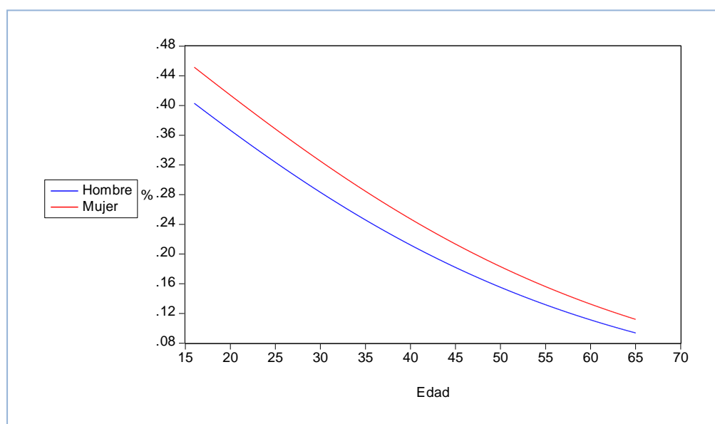
Gráfico 5.1: Curva de respuesta de la edad y el sexo
