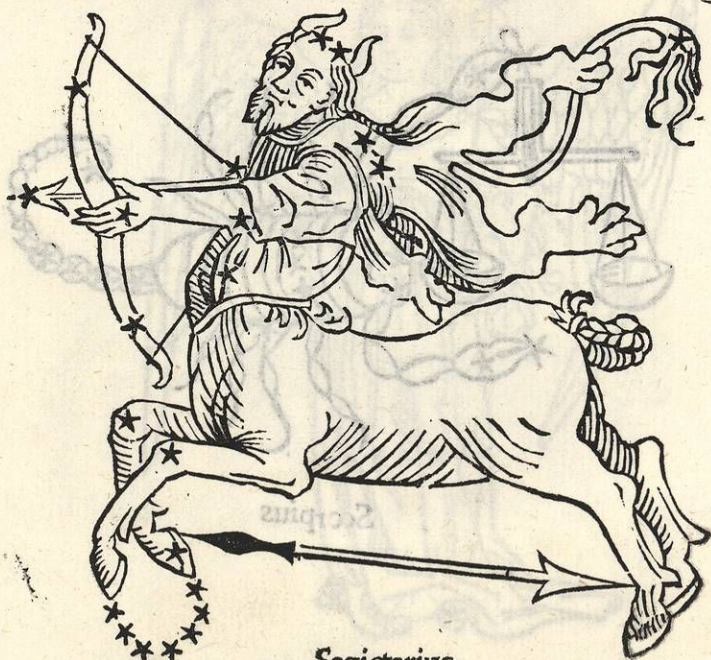
Sagictarius
