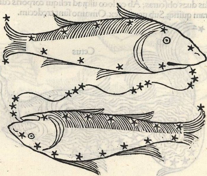
Pisces
