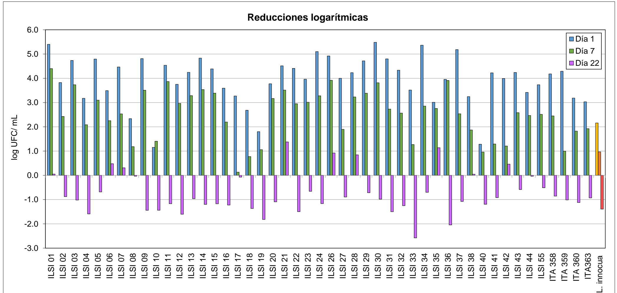
Figura 4. Reducciones logarítmicas para todas las cepas Listeria monocytogenes y una cepa de Listeria innocua tras un tratamiento de HPP ( 500 MPa 1 min) a día 1, a día 7 y día 22 a pH 6.
