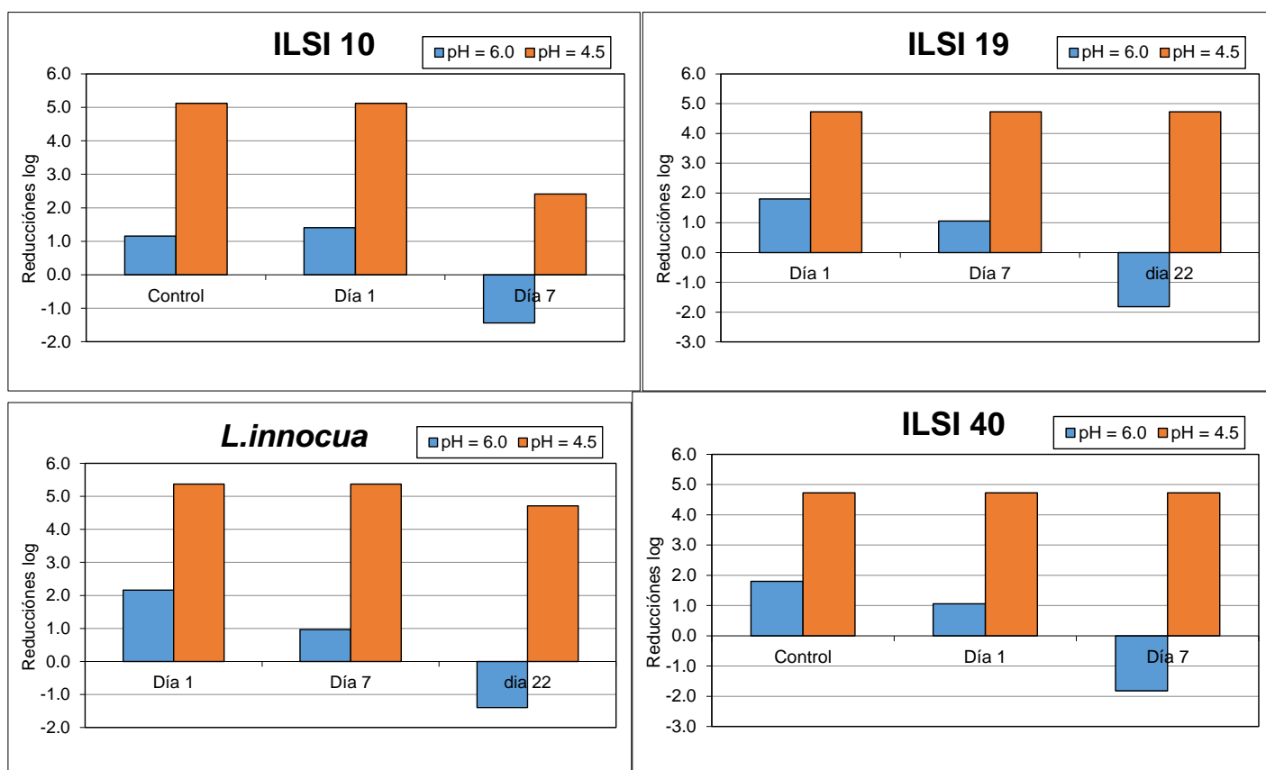
Figura 8. Reducciones logarítmicas para las cinco cepas seleccionadas como más resistentes a día 1, día 7 y día 22 a pH 6 y a pH 4.5
