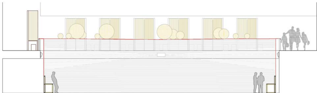
SECCIÓN LONGITUDINAL
