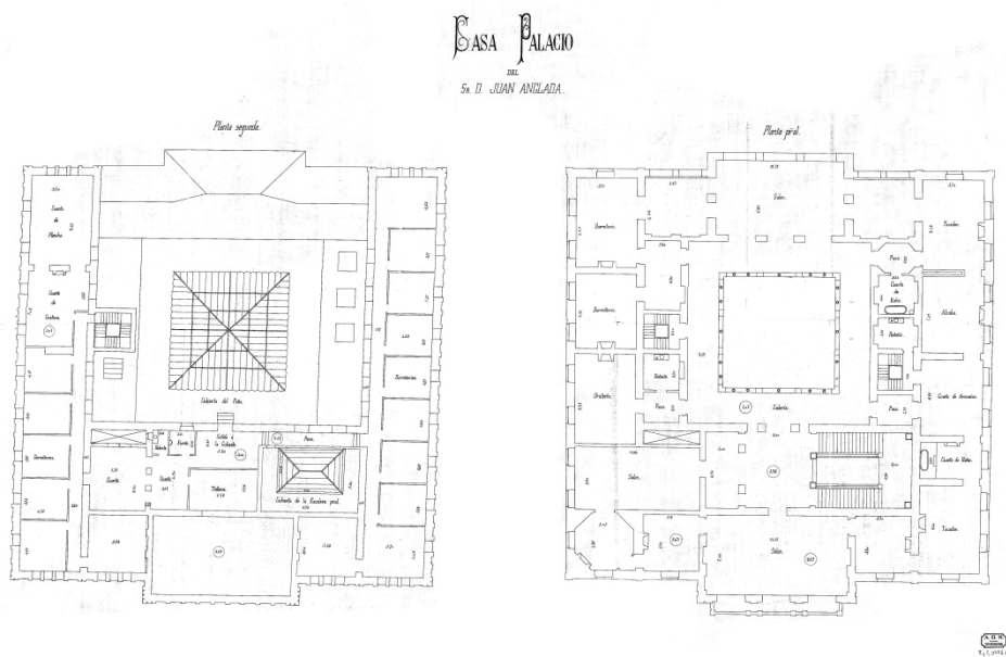
Fig. 7: Plano de la planta principal y ático, AHN Madrid. Diversos_Titulos_Familias 3773, exp. 6.
