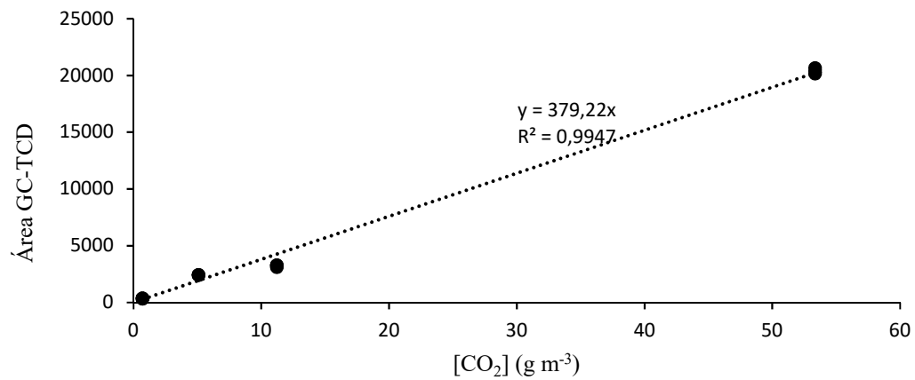
Figura 20. Recta de calibración de la concentración de CO 2 (22/6/2015).
