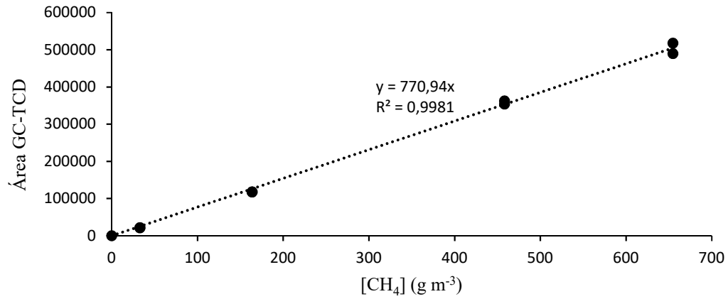
Figura 19. Recta de calibración de la concentración de CH 4 (22/6/2015).
