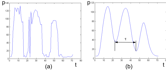
Fig. 8. (a) Variación de la distancia entre los pies en píxeles p en el eje de ordenadas a lo largo de los fotogramas (tiempo t en el eje de abscisas) y (b) suavizado de la curva de distancia ( Nota : los valores de las distancias representadas son previos a la normalización).
