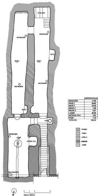
Fig. 4. Plano de levantamiento de bodegas en Torquemada. Ficha Bodega (L.14.16) Barrio de Ladredo, calle Mazuela, bodega nº 16. Fuente: los autores.
