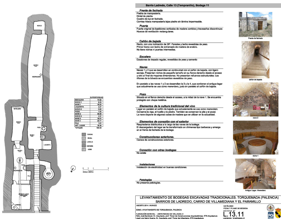
Fig. 5. Plano de levantamiento de bodegas en Torquemada. Ficha Bodega (L.13.11) Barrio de Ladredo, calle Tempranillo, bodega nº 11. Fuente: los autores.
