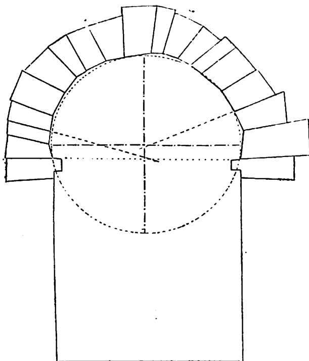
Fig. 2. Arco de la portada.
