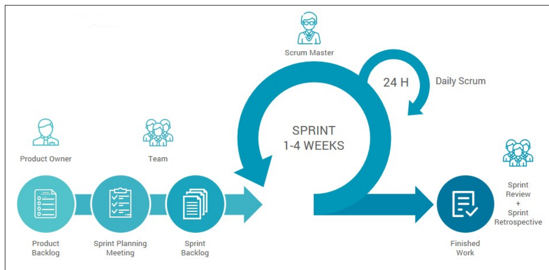
Figura 2.1: Proceso Scrum
