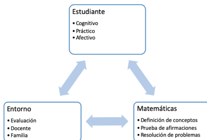
Figura 1. Modelo propuesto
