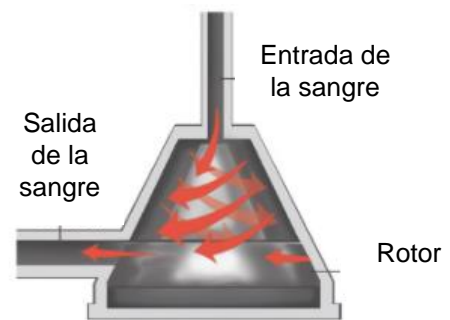
Figura 4. Bomba de flujo centrífugo. Fuente: Modificada a partir de la fuente bibliográfica (11).
