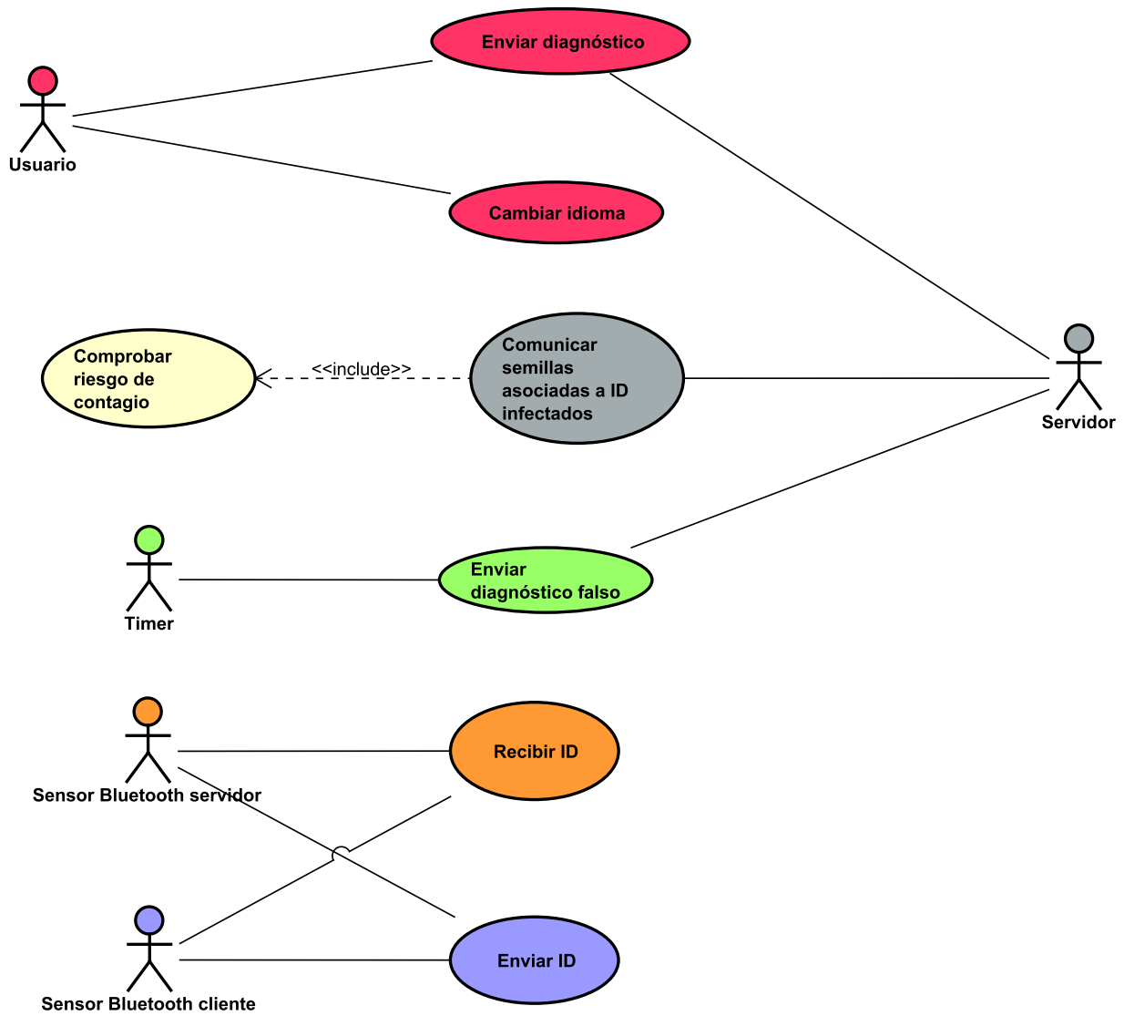
Figura 7: Diagrama de casos de uso
