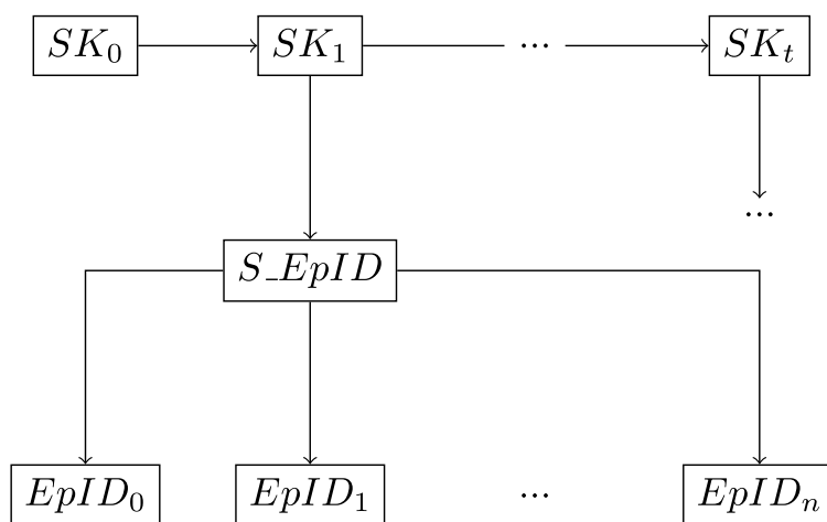
Figura 8: Esquema de generación de identificadores efímeros
