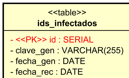
Figura 12: Modelo físico de la base de datos del servidor
