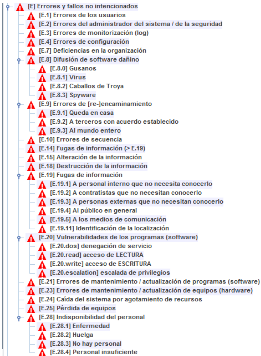
Figura 47: Listado de amenazas de PILAR Basic (Parte 3)
