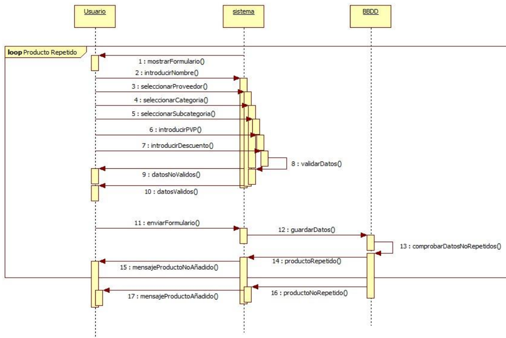
Ilustración 16 - Caso de Uso: Crear nuevo producto
