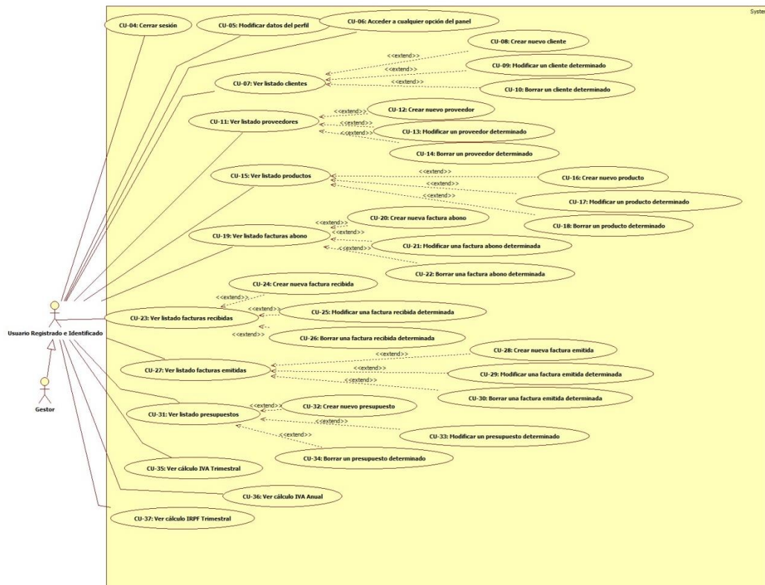
Ilustración 10 - Caso de Uso: Usuario Gestor
