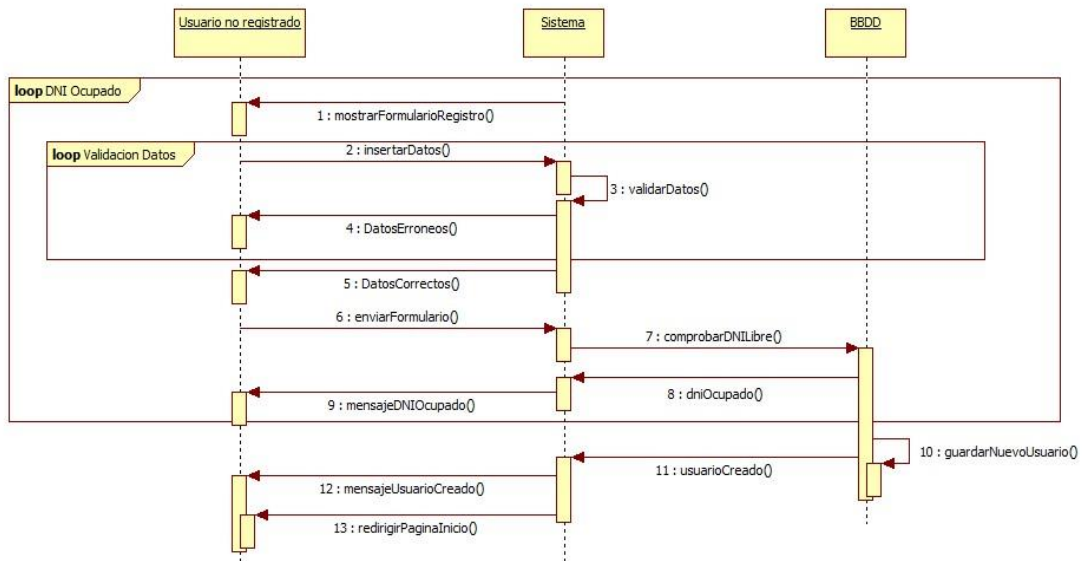
Ilustración 15 - Caso de Uso: Registrarse en la aplicación
