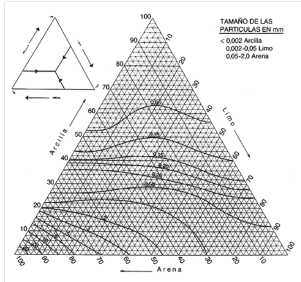
Figura 9. Diagrama textural para la determinación de la conductividad hidráulica a saturación ( K_{sat} en cm \cdot h^{-1} ) (López Cadenas, 1998). Los datos texturales de entrada deben ser los del horizonte menos permeable.
