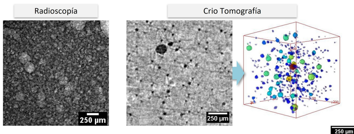
Figura 0-14: Ejemplo de la estructura celular a tiempos cortos de rección obtenida mediante Radioscopia y Crio-Tomografía.
