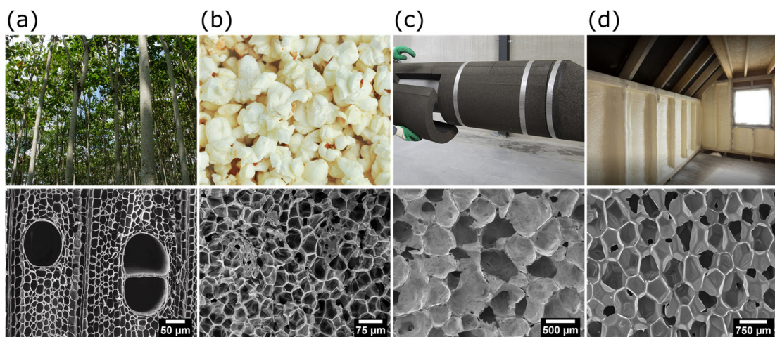
Figura 0-1: Estructura celular característica de (a) la madera de balsa, (b) las palomitas de maíz, (c) las espumas de vidrio y (d) el aislamiento de espuma de poliuretano.
