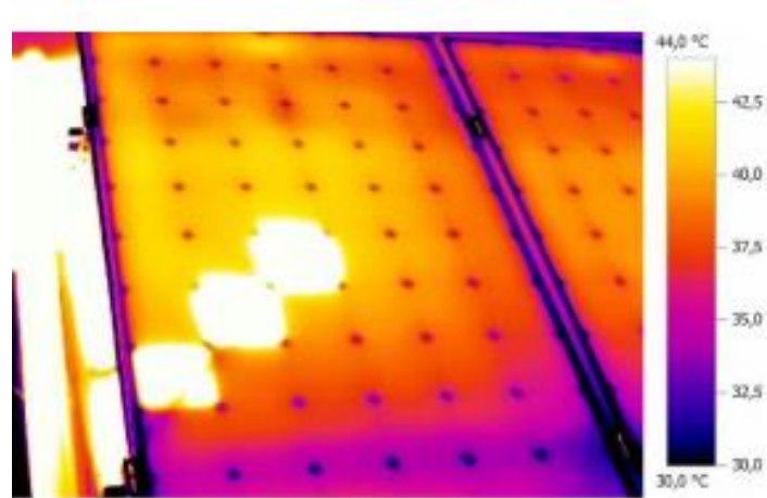
Figura 20: Efecto hotspot en cámara termográfica. Fuente: Amara Energy Transition
