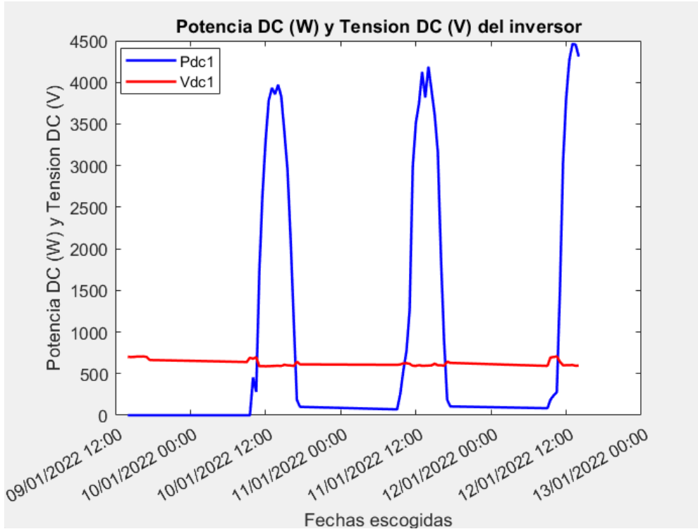
Figura 65: Potencia y tensión en continua. Fuente: Elaboración propia.
