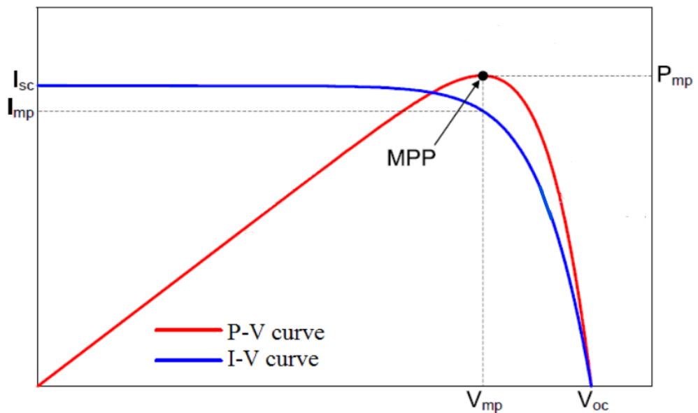
Figura 16: Curva característica I-V y P-V con representación del Pmpp. Fuente: Buscador de Google
