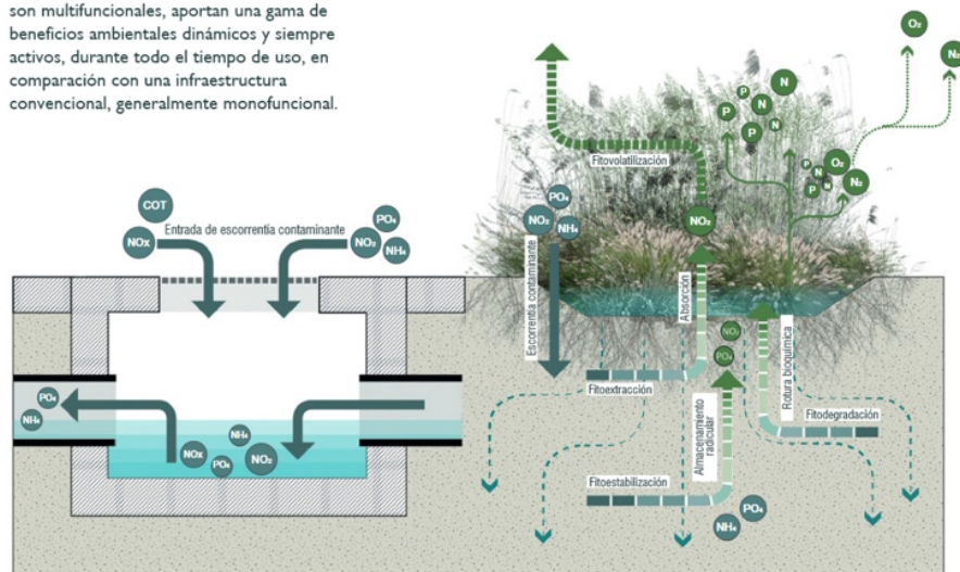
Fig. 4. Comparación entre un sistema de eliminación de aguas de lluvia convencional y un SUDS. Fuente: Claudia Sánchez Escudero (UVa), a partir de Montlleó y Spanou (2022).
