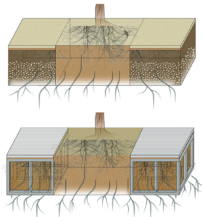
Fig. 9. Propuestas de suelo estructural para alcórcos. Arriba: suelo estructural con gravas. Abajo: suelo estructural con celdas. Ambas permiten un correcto desarrollo radicular. Fuente: Montlleò y Spanou (2022).
