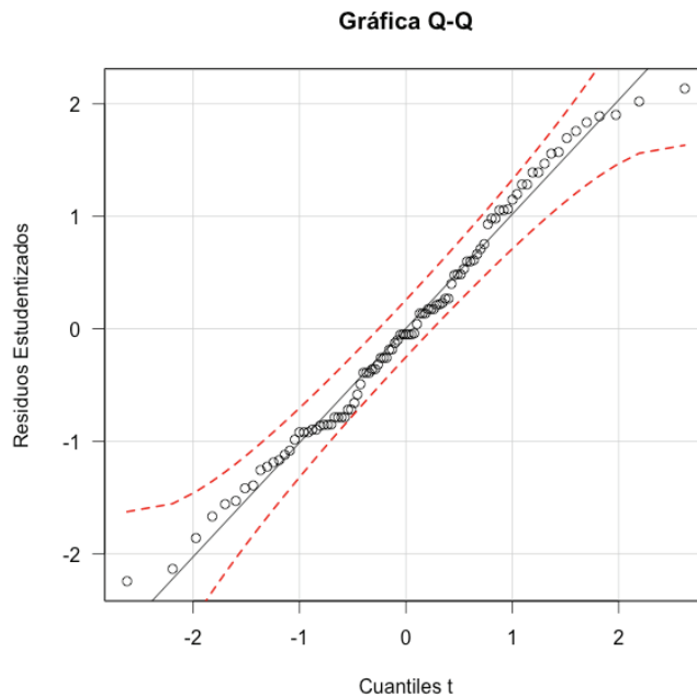
Figura 1. Gráfica Q-Q
