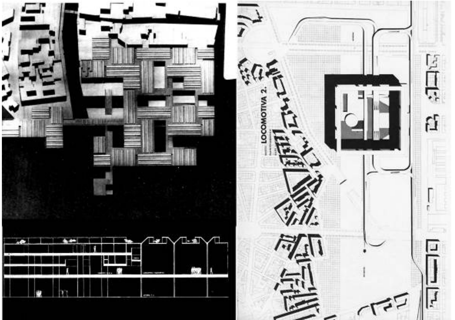
[Fig. 7]. a) LC: Hospital de Venecia, 1964-65. Detalle de la sección, incluyendo laboratorios, conduits y rampas de conexión entre niveles superiores. b) LC: Hospital de Venecia; maqueta del 2º proyecto, 1965, vista cenital. c) G. Polesello, A. Rossi, L. Meda. Proyecto para el Centro direccional de Turín, 1962. Fuente: a) Sarkis, Le Corbusier's Venice Hospital and the mat building revival , 4. b) Le Corbusier, Oeuvre Complète , vol 7, 141. c) Piperno, "Grandi concorsi italiani tra il 1945 y 1984", 14.
