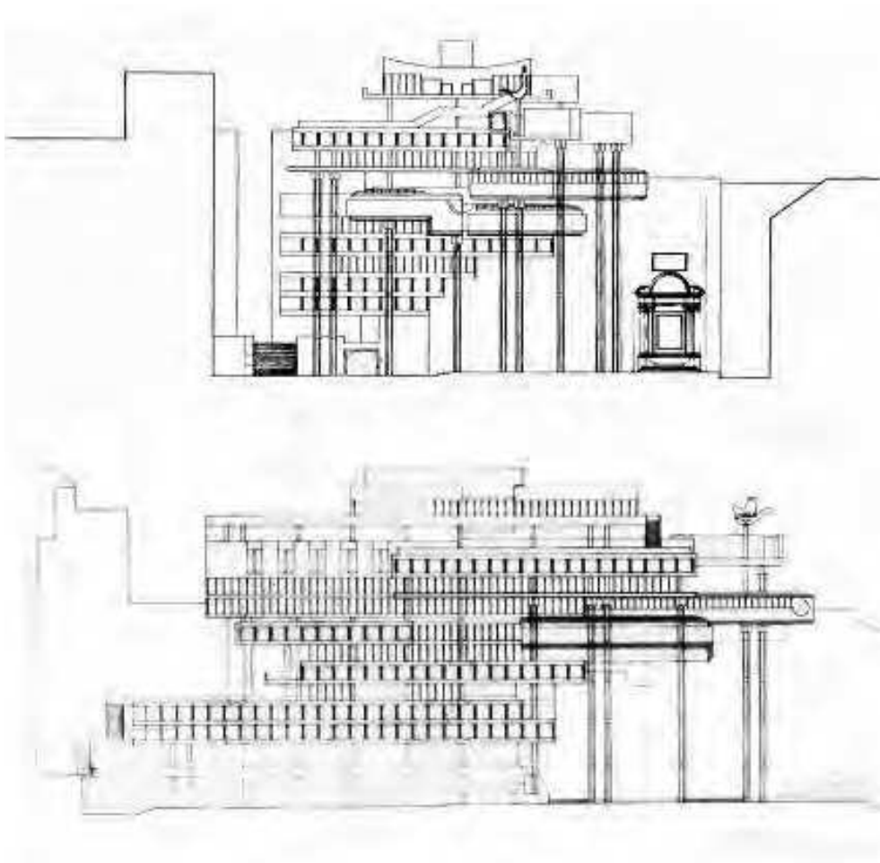
[Fig. 10]. Alzados norte y este, con indicación de las conexiones entre terrazas mediante escaleras exteriores: plantas primeras y plantas superiores con el restaurante. Fuente: Tafuri, Il Concorso per i nuovi uffici della Camera dei Deputati , 103.
