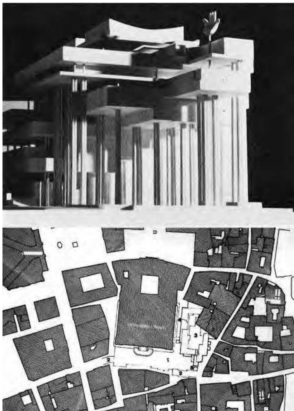
[Fig. 1]. Maqueta y planta de situación, orientada al sur. 1. Plaza del Parlamento; 2. Entradas al parking; 3. Nuevo edificio. 4. Terraza que coge la cota de la plaza de Montecitorio. Fuente: Aymonino, Giuseppe Samonà. Cinquante ans d'architecture , 123; Tafuri, Il Concorso per i nuovi uffici della Camera dei Deputati , 99.
