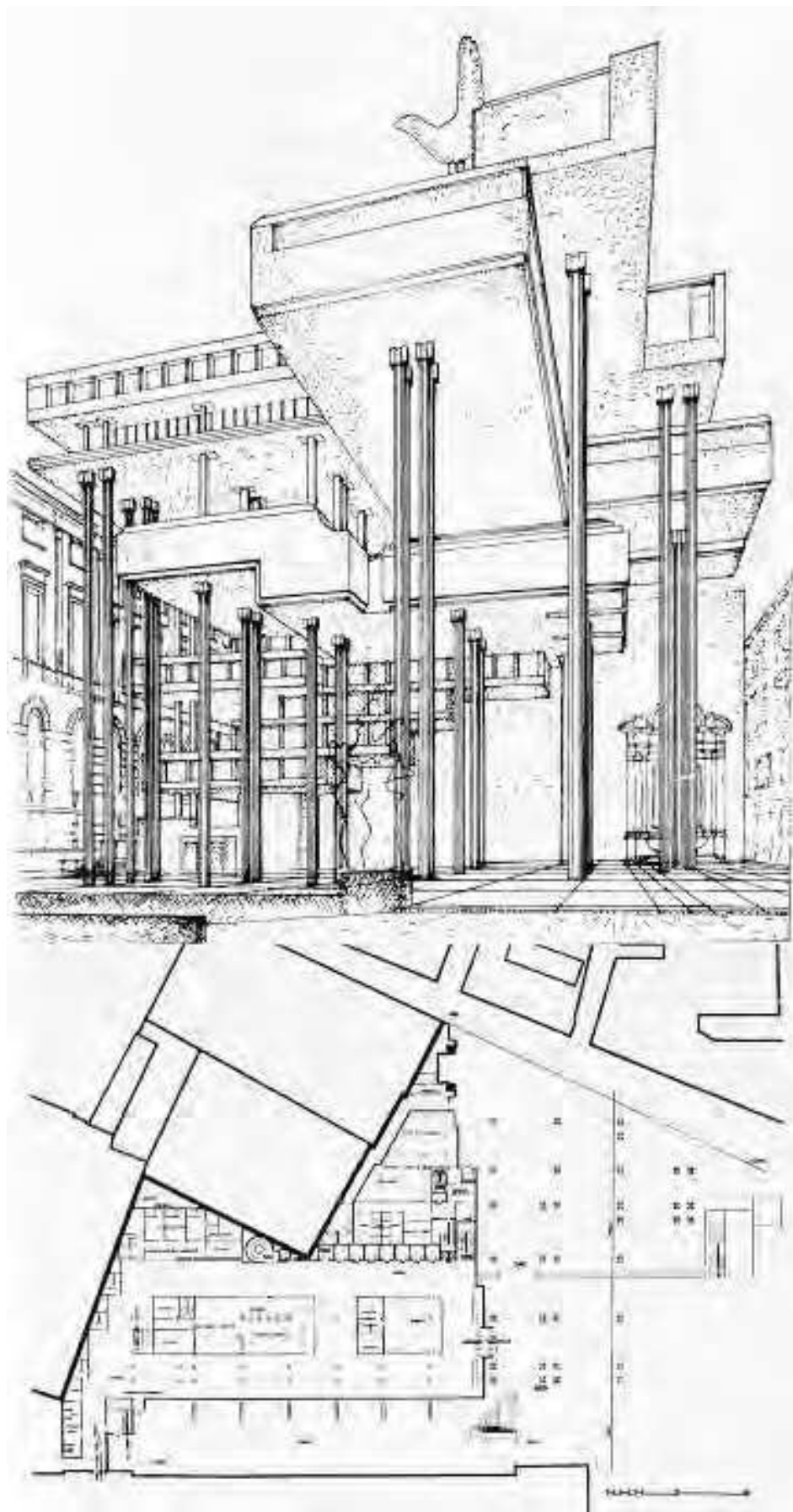
[Fig. 3]. Vista desde el norte, con la entrada al parking en primer plano, y Planta baja a cota \pm 0,00 . Materiales: pilares metálicos, agrupados de 4 en 4 y solidarizados cada 5 metros; travertino en fachadas, colocado entre impostas de cobre. Fuente: Bonfanti, Arquitectura Racional , 97; Samonà, L'Unità Architettura Urbanistica , 593.
