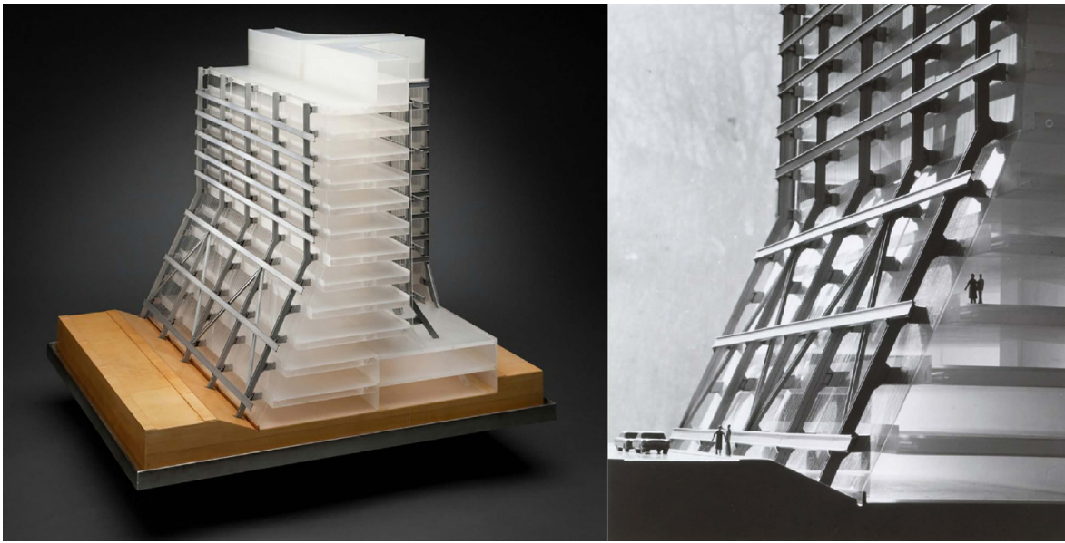
Figura 8. J. Stirling, maqueta de la sección de un módulo de la sede de Dorman Long, Middlesbrough (Reino Unido), 1965; realizada para la presentación del proyecto (impresión en gelatina de plata, 16,7x24,6 cm).
