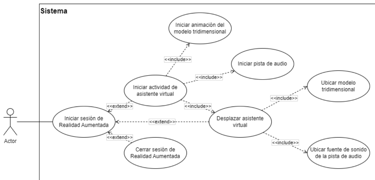
Figura 3.1: Diagrama de casos de uso
