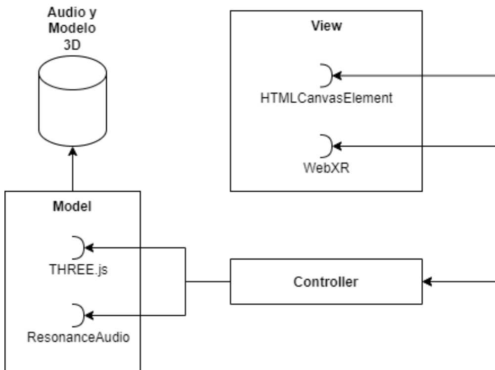
Figura 3.4: Diagrama de componentes
