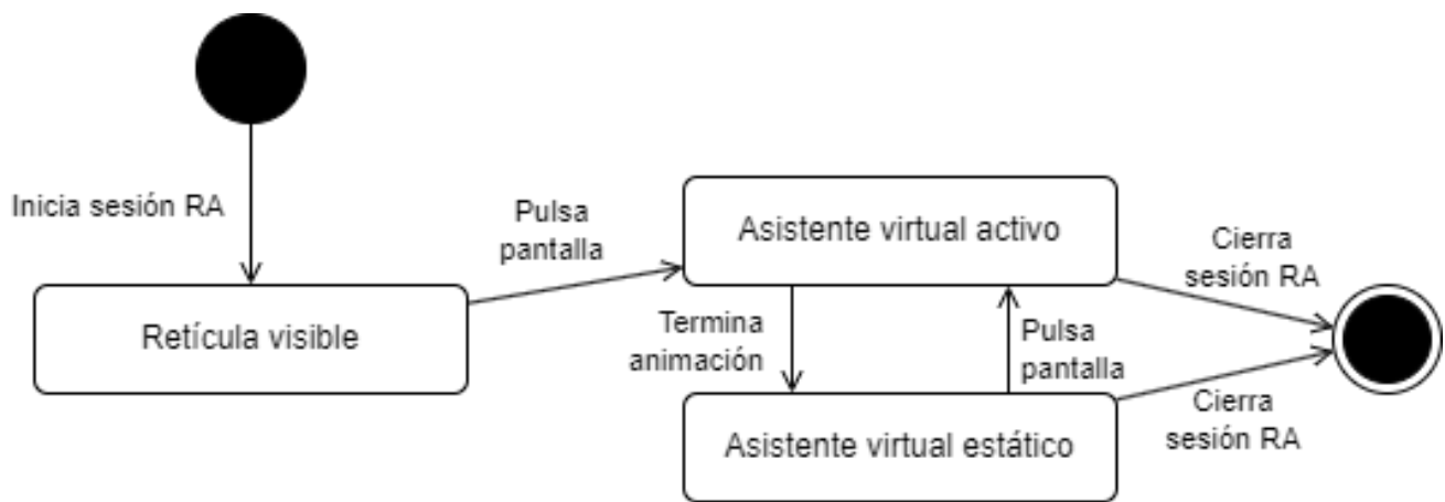
Figura 3.6: Diagrama de máquinas de estado
