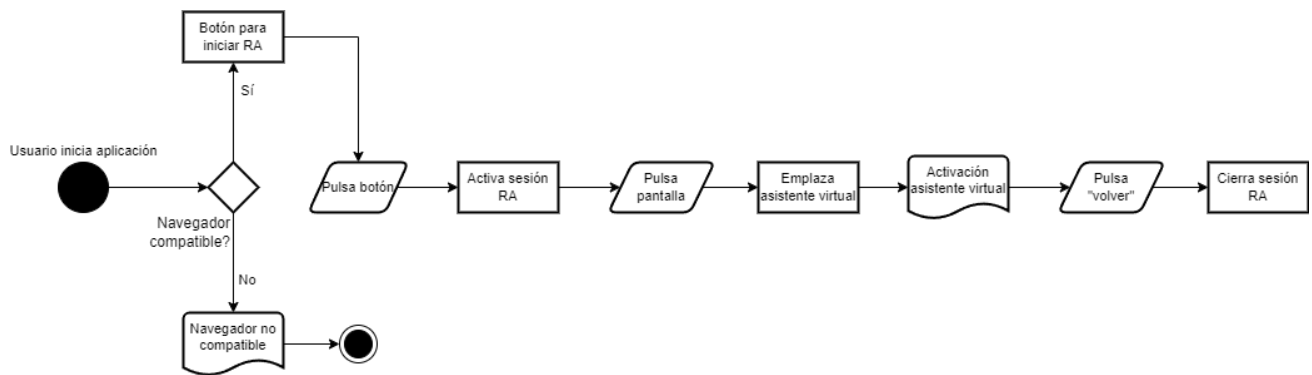
Figura 3.7: Diagrama de actividades
