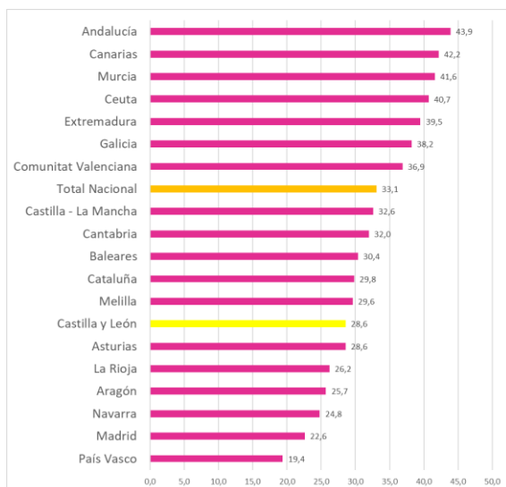
Ilustración 12: Carencia material en el año 2023 por CCAA
