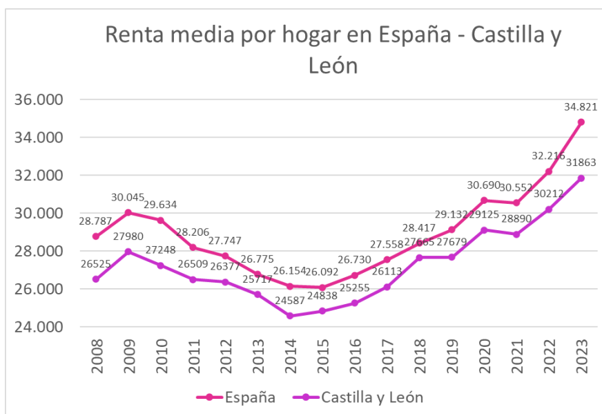
Ilustración 1: Renta media por hogar. España y Castilla y León
