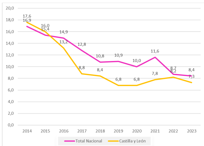
Ilustración 14: Viviendo en hogares con baja intensidad en el trabajo (0 a 64 años). España.
