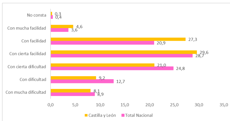
Ilustración 15: Hogares según dificultades para llegar a fin de mes. 2023.
