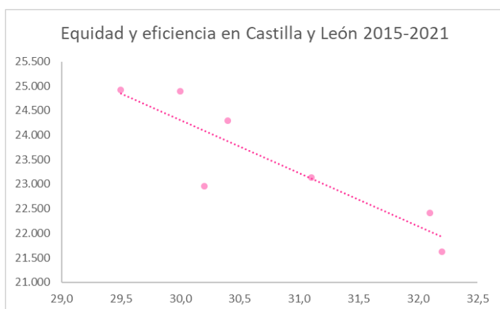
Ilustración 23: Equidad y Eficiencia en Castilla y León. Evolución 2015-2021.
