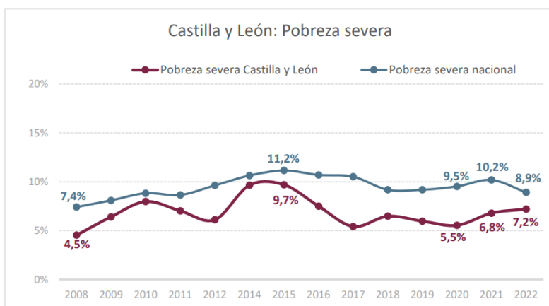
Ilustración 8: Pobreza severa en Castilla y León-Total Nacional.
