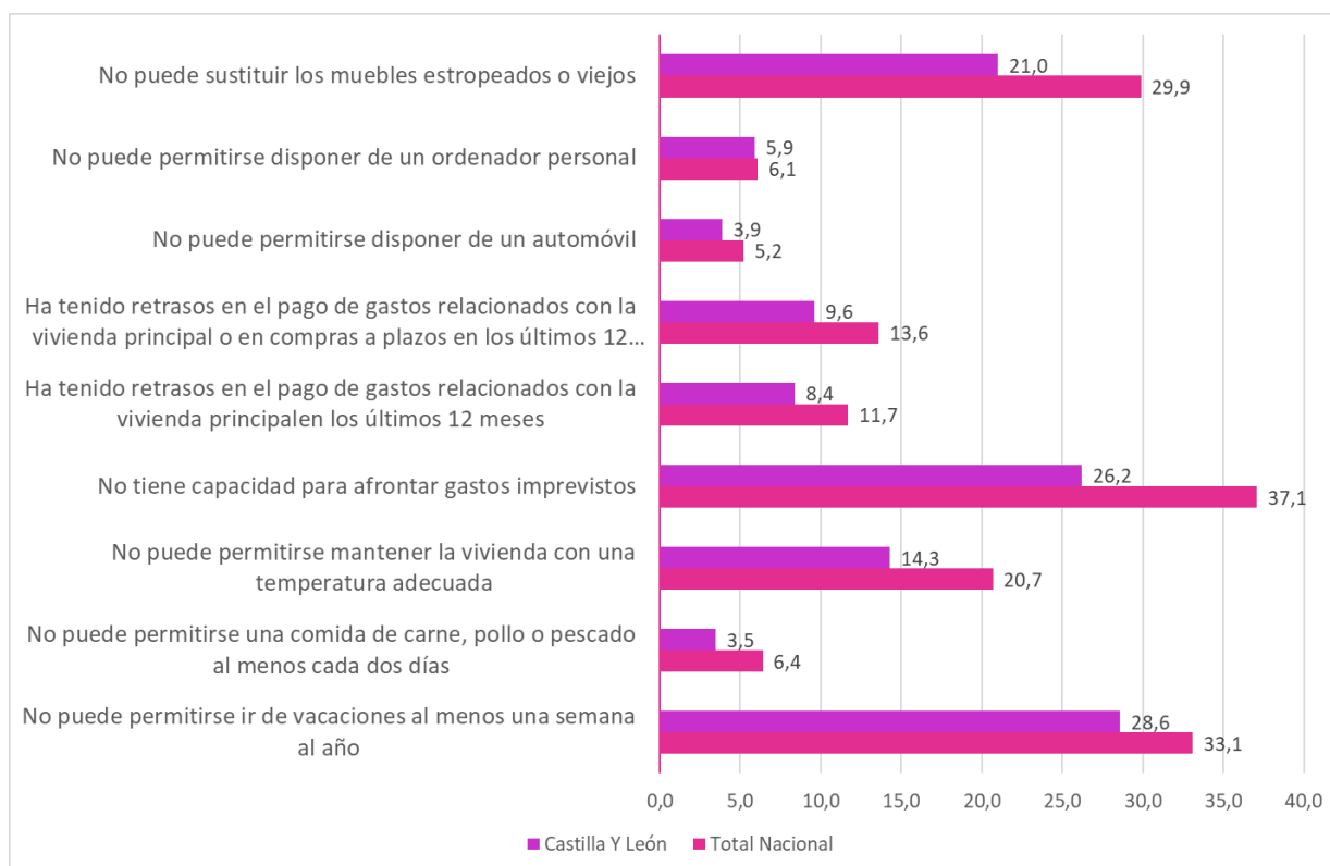
Ilustración 13: Carencia material Castilla y León – Total nacional. Por tipos.
