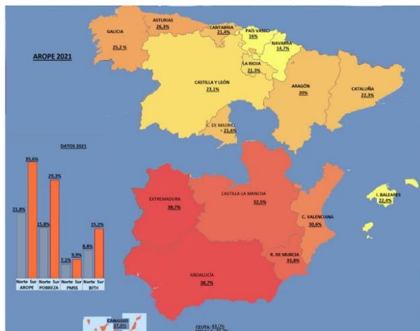
Ilustración 3: Distribución territorial de AROPE en el año 2021
