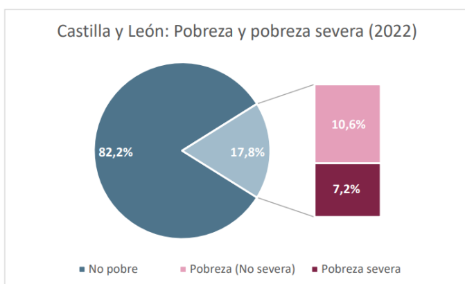
Ilustración 9: Pobreza severa en Castilla y León
