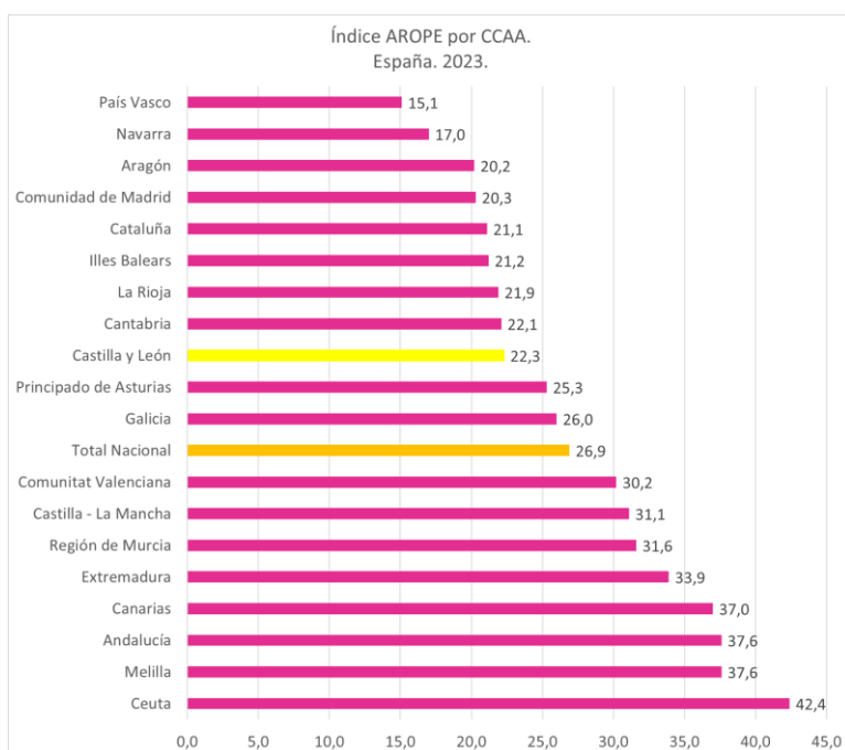
Ilustración 5: Índice AROPE 2023 por CCAA
