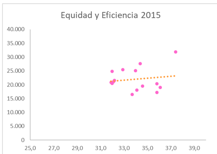
Ilustración 19: Equidad y eficiencia en el año 2015.
