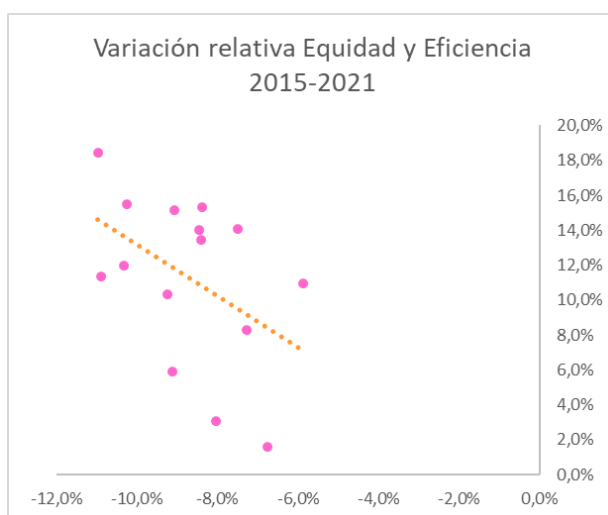
Ilustración 22: Equidad y eficiencia en el período 2015-2021. Rel.
