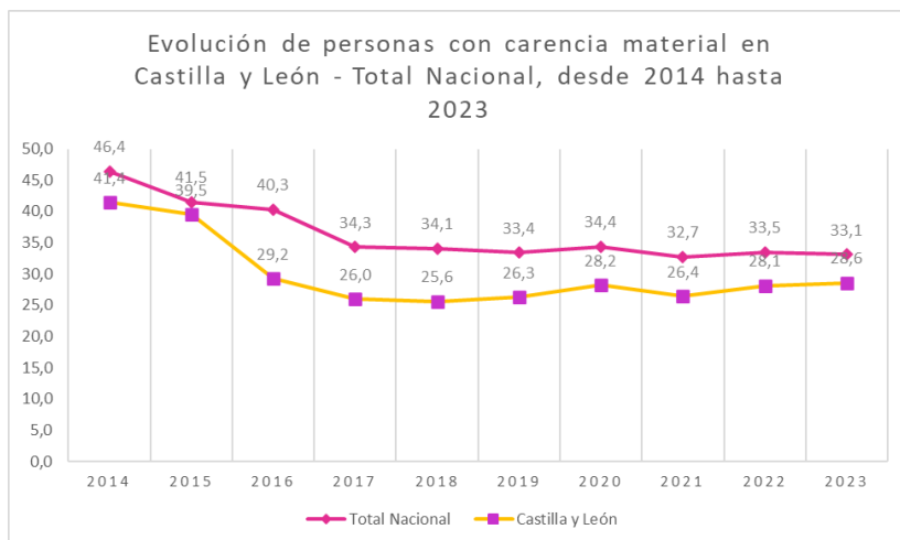
Ilustración 11: Porcentaje de población con carencia material.
