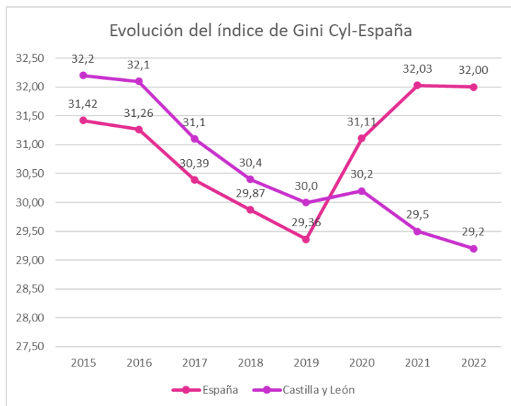
Ilustración 17: Evolución del índice de Gini. Castilla y León- España.
