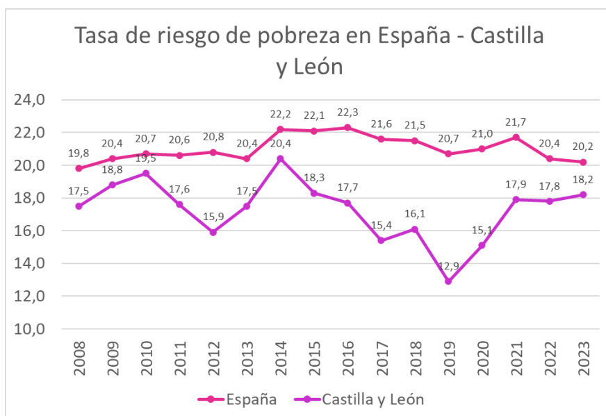
Ilustración 2: Tasa de riesgo de pobreza. España y Castilla y León
