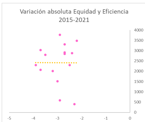
Ilustración 21: Equidad y eficiencia en el período 2015-2021. Abs.
