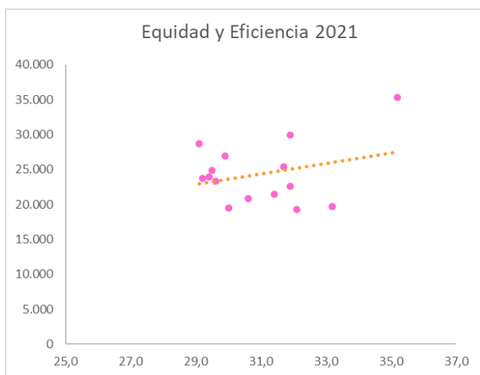
Ilustración 20: Equidad y eficiencia en el año 2021.
