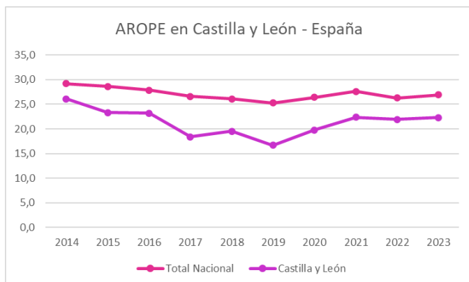
Ilustración 4: Evolución AROPE. Castilla y León – España.
