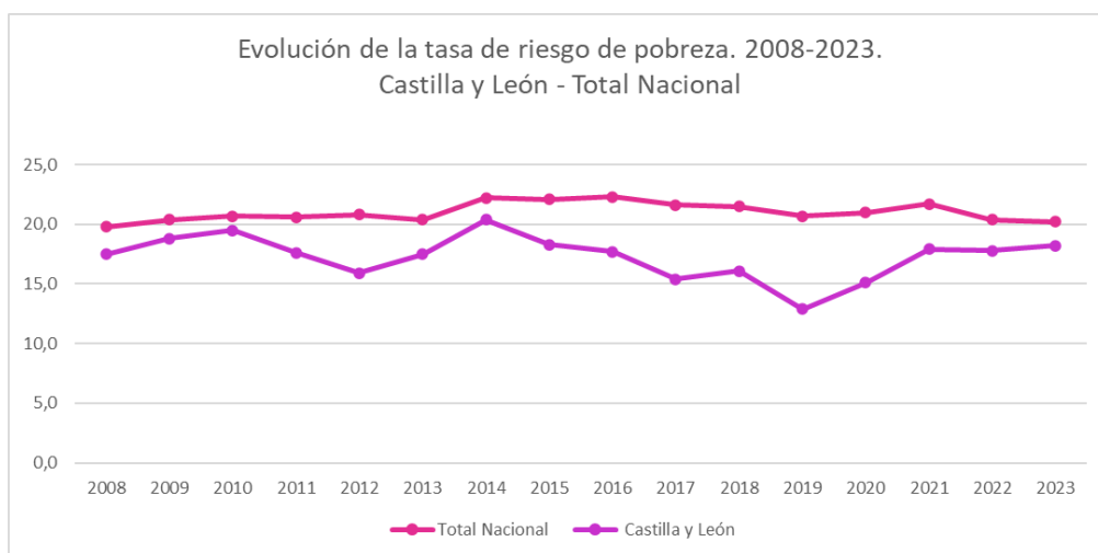
Ilustración 6: Evolución de la tasa de riesgo de pobreza. 2008-2023.
