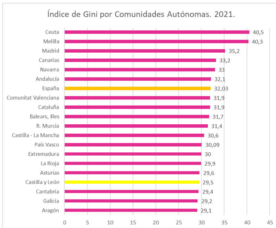
Ilustración 18: índice de Gini por Comunidades autónomas. 2021.
