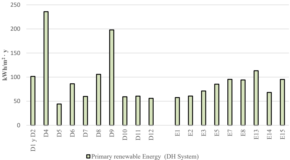
Fig. 12. EI_{pr} DHS (kWh/m²·y).
