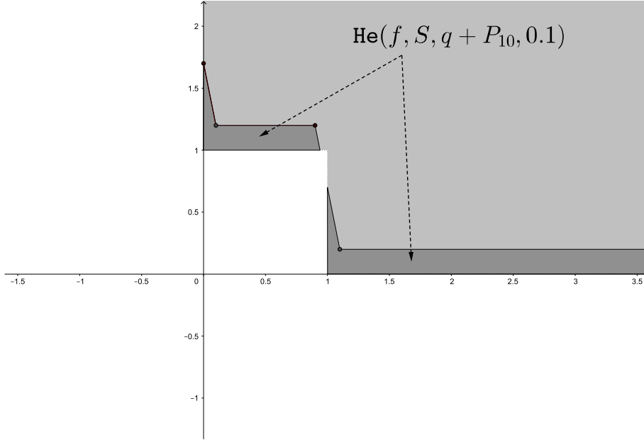
FIG. 2. \text{He}(f, S, q + P_{10}, 0.1)
