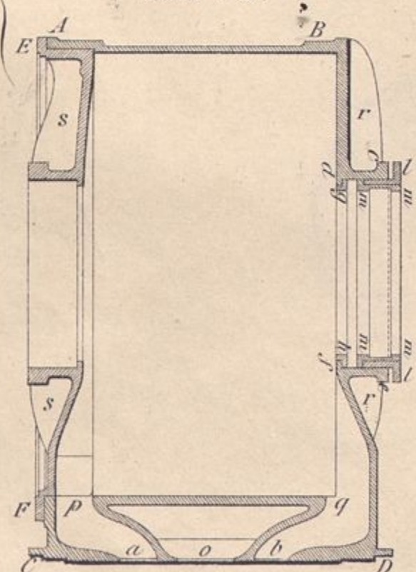
Corte CD.
