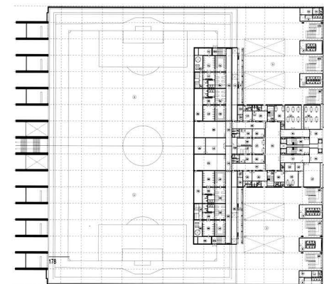
PLANTA SÓTANO
