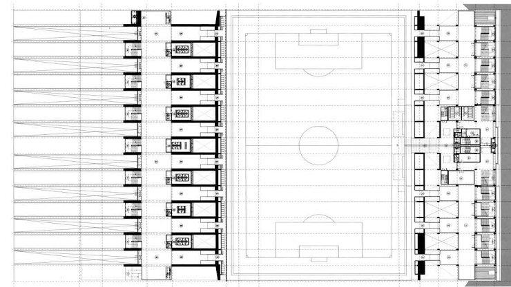
PLANTA ACCESO
