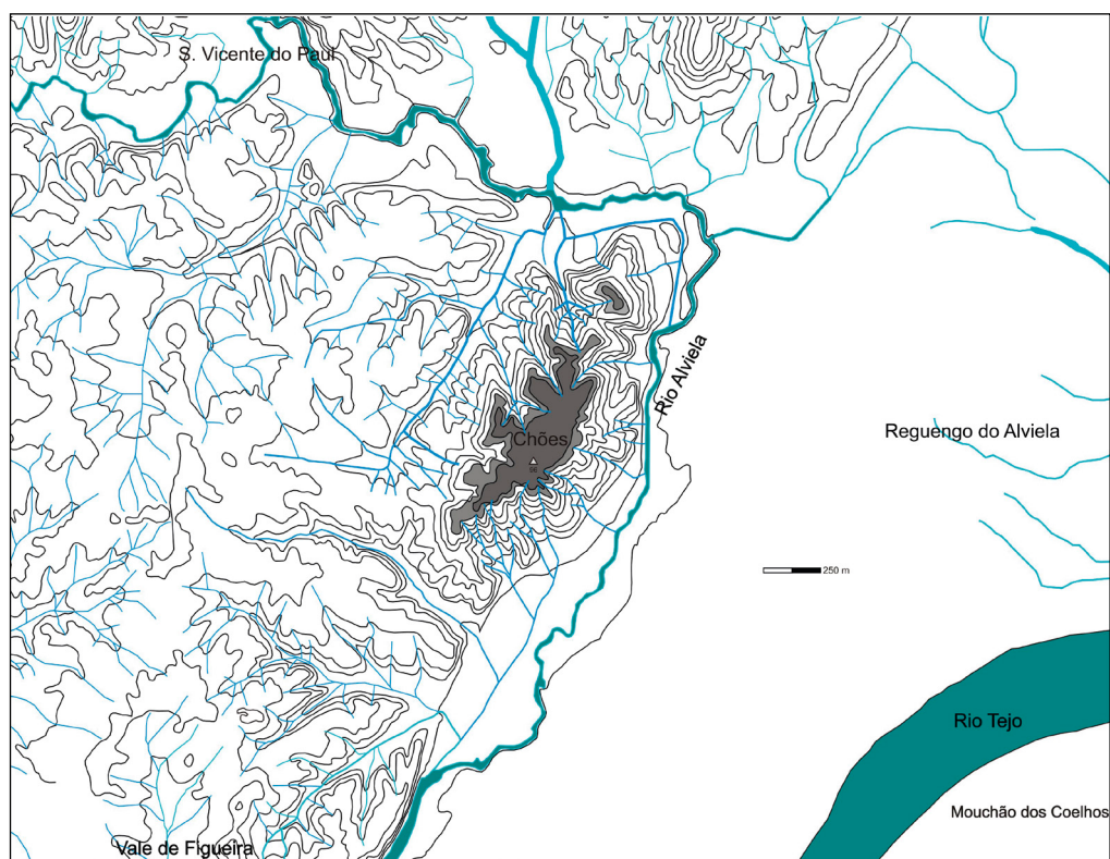
Figura 2. Planta da área de Chões de Alampé, com as curvas de nível e localização das linhas de água produzida a partir da carta militar 1:25.000, folha n.º 341 de 1969. Área de dispersão de materiais assinalada a cinzento
