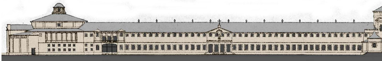
Fig. 219 Alzado meridional de la Universidad Laboral.
