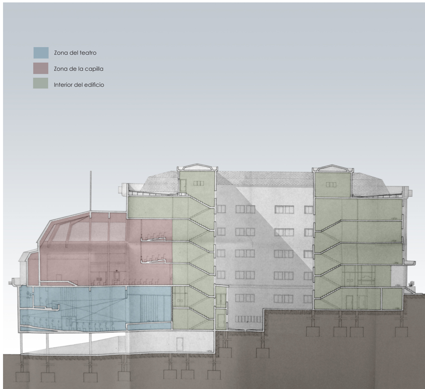
Fig. 311 Sección transversal de la residencia de ancianos «Reina de la Paz» según el proyecto de 1973.
