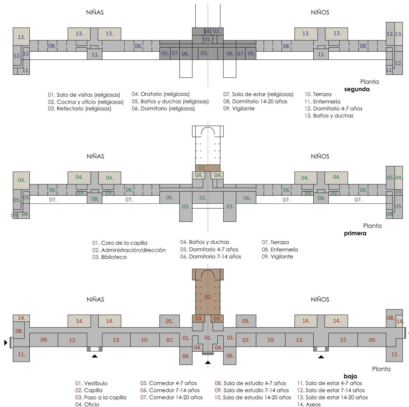
Fig. 37 Plantas del colegio-orfanato Nuestra Señora del Tránsito en 1973-1998.
