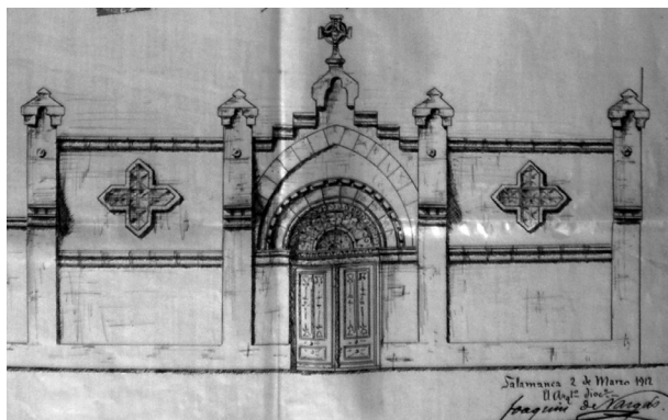
Fig. 102 Alzado de la capilla hacia la calle San Martín. 1912.
