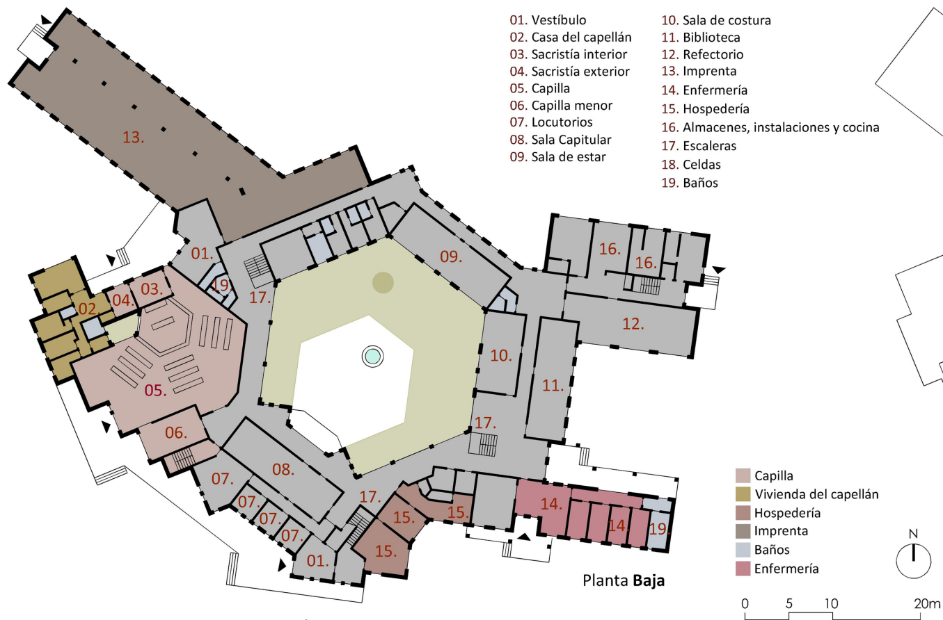
Fig. 278 Plantas del monasterio de la Ascensión del Señor.
