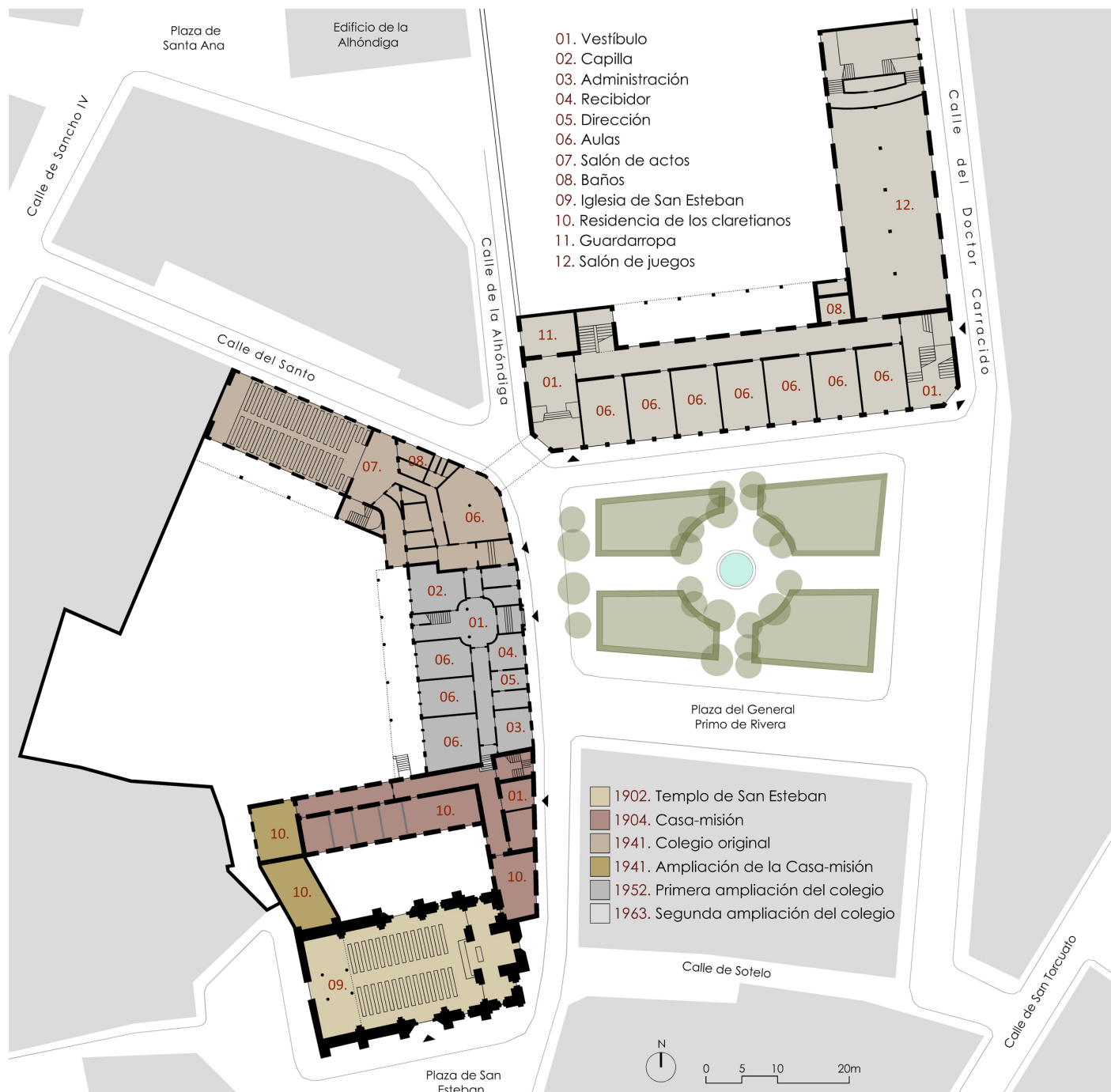
Fig. 170 Planta baja del colegio Corazón de María tras la última ampliación, lo que coincidiría con el período 1963-1980.
