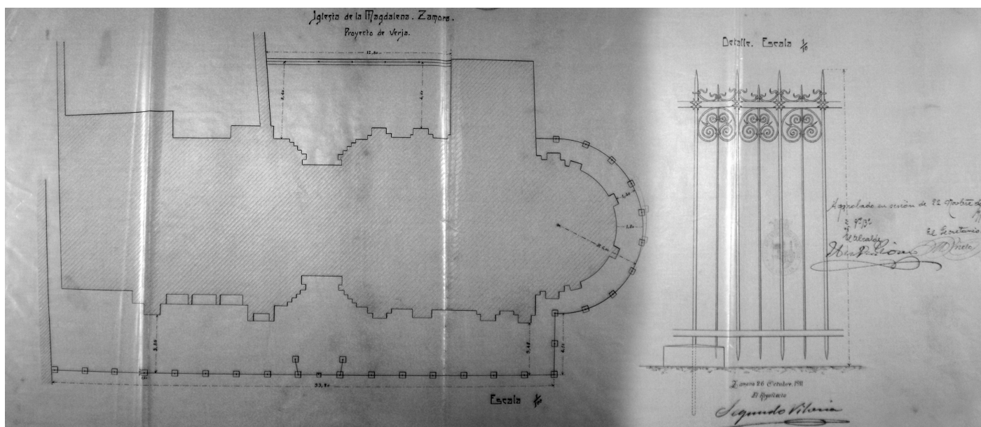
Fig. 159 Proyecto de 1911 para la verja de la iglesia de la Magdalena. Arquitecto Segundo Viloria.
