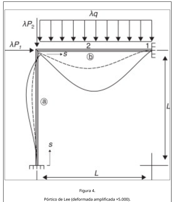
Figura 4. Pórtico de Lee (deformada ampliada \times 5.000 ).
