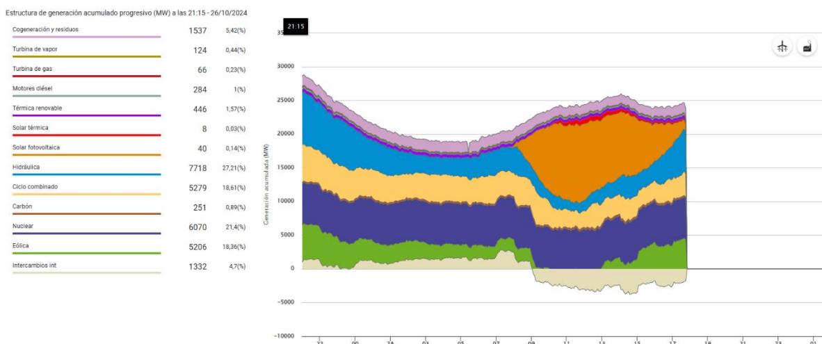
Figura 17. Generación de energía por tipo de generación y por horas en España sen REE
