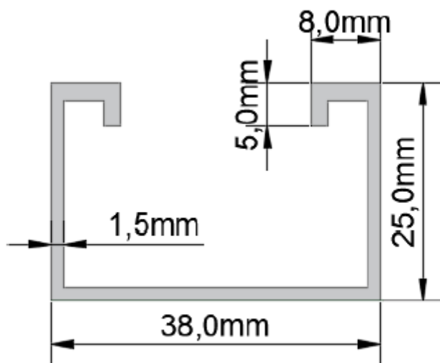
Figura 14. Dimensiones estructura de soporte a utilizar para instalar los módulos fotovoltaicos
