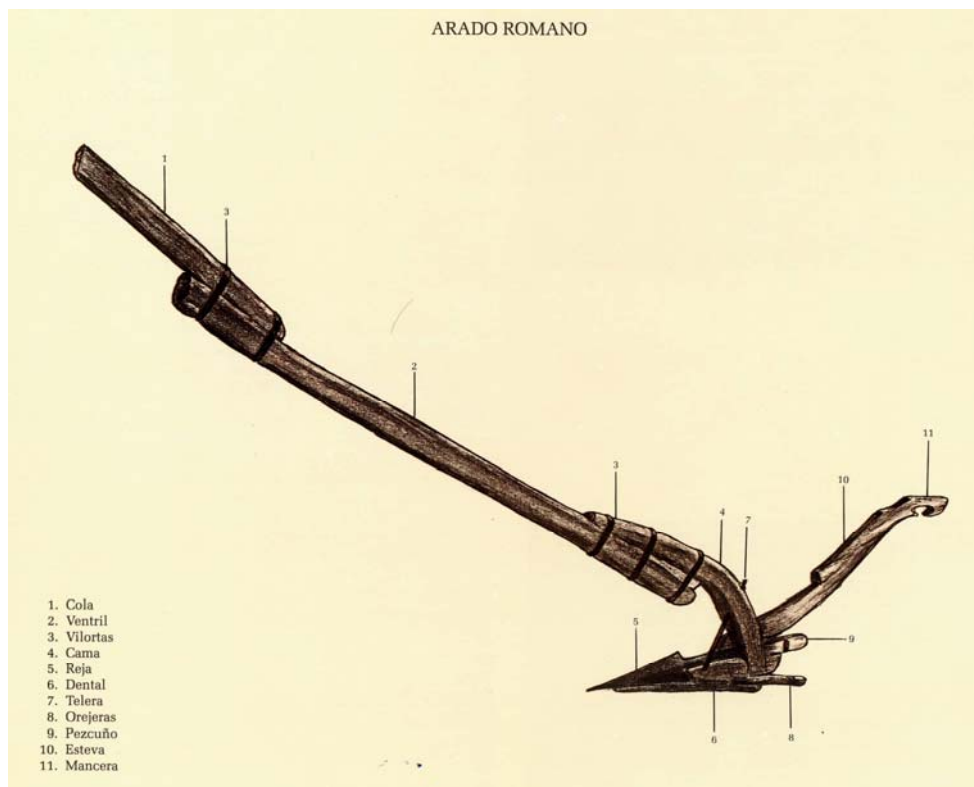
Partes del arado romano 27
