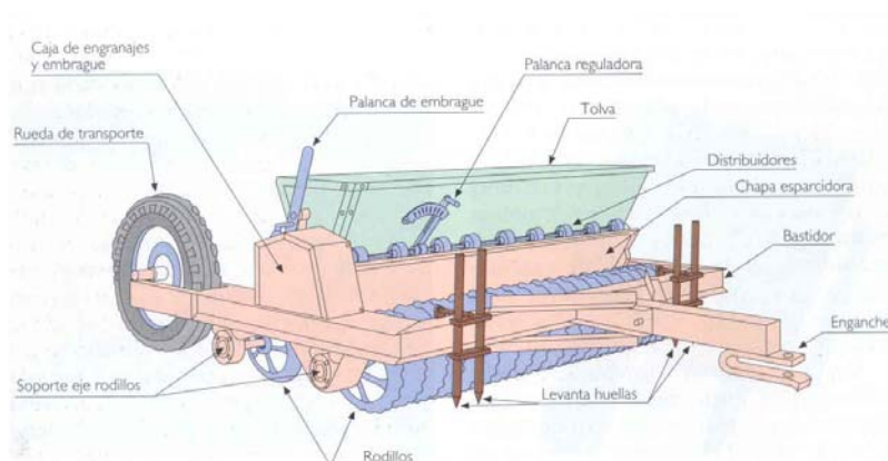
Sembradora a voleo 22
