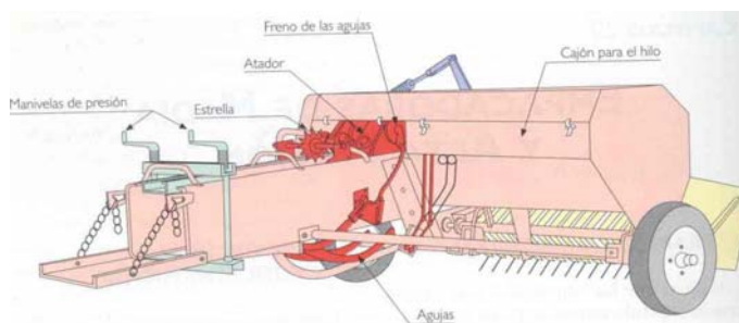
Vista posterior de una empacadora 10
