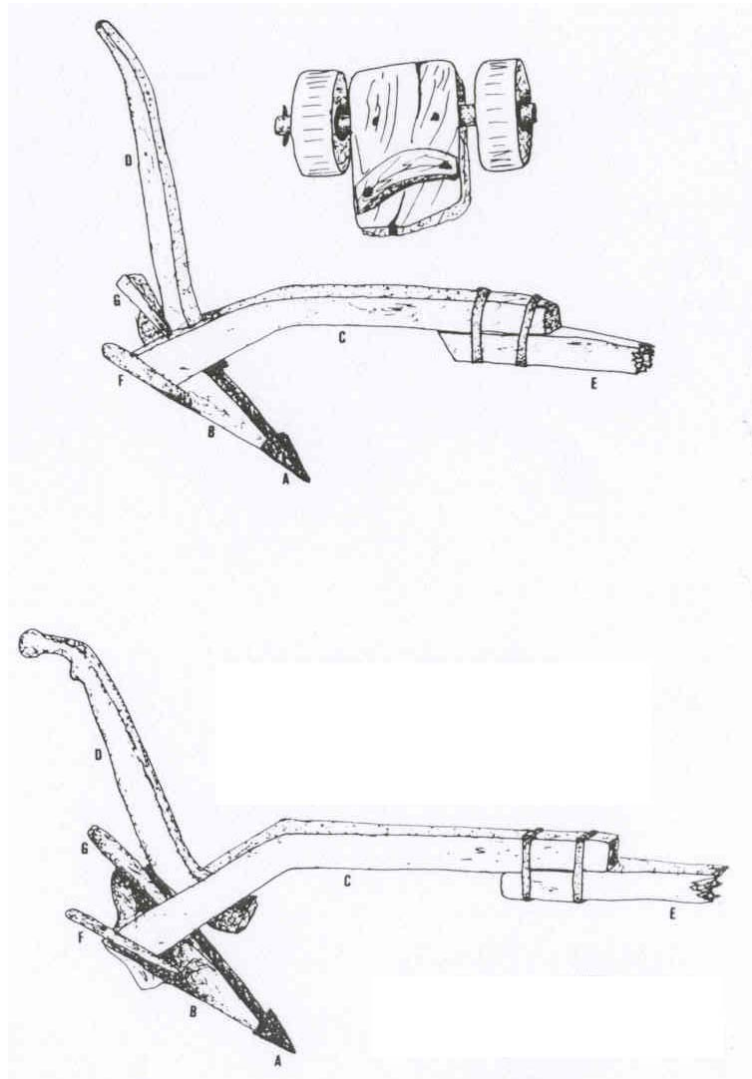
Partes del arado 47
