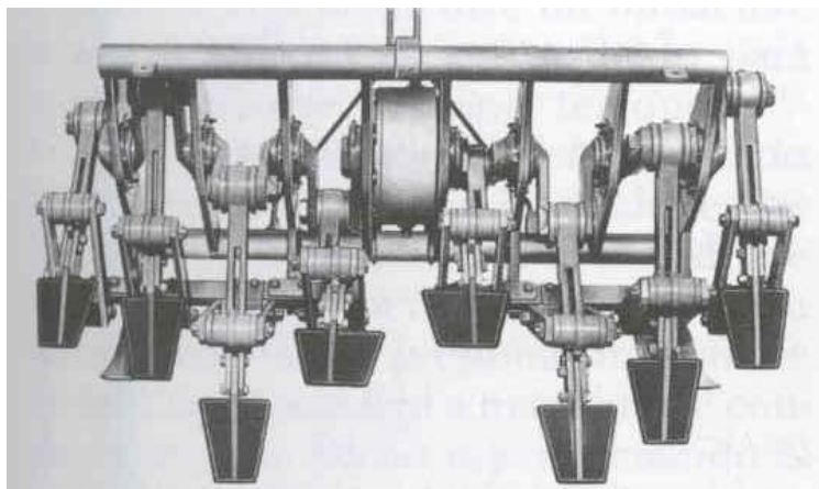
Vista posterior de una azada mecánica 51
