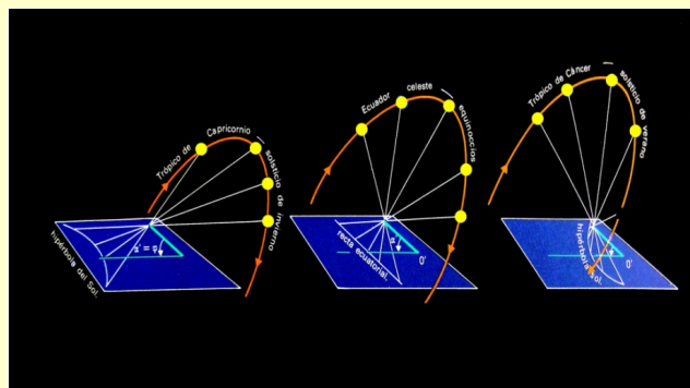
Fig. 7. Ilustración del fundamento astronómico de la meridiana
