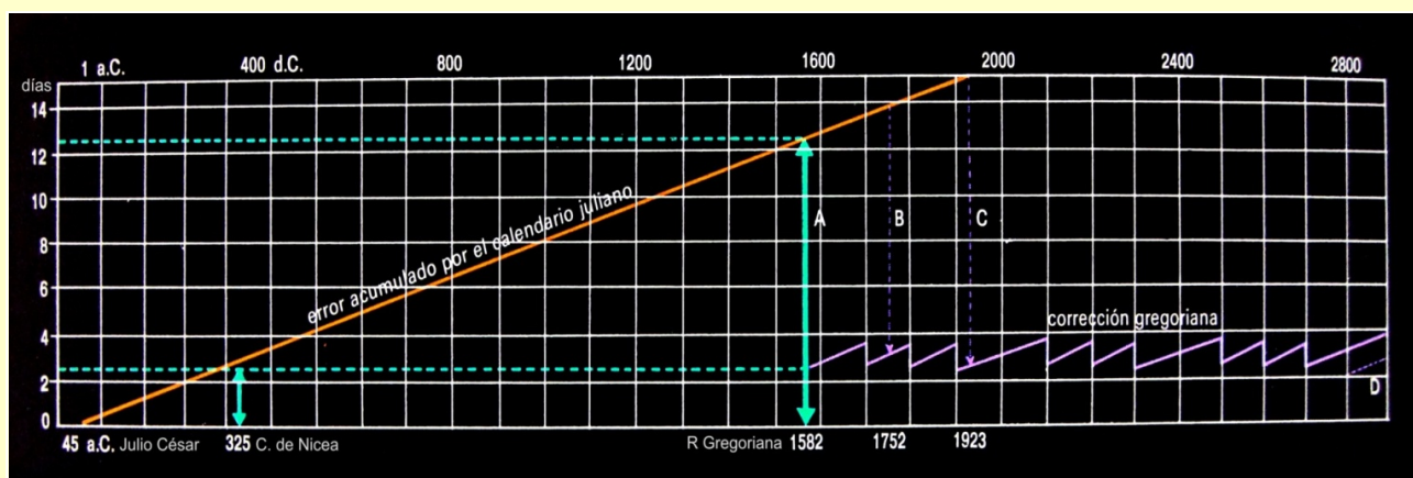
Fig. 6. Esquema de la corrección introducida por el calendario gregoriano.
