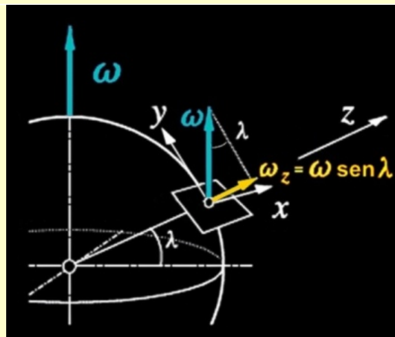
Fig. 9. Esquema de la descomposición de la velocidad de rotación terrestre en función de la latitud del lugar
