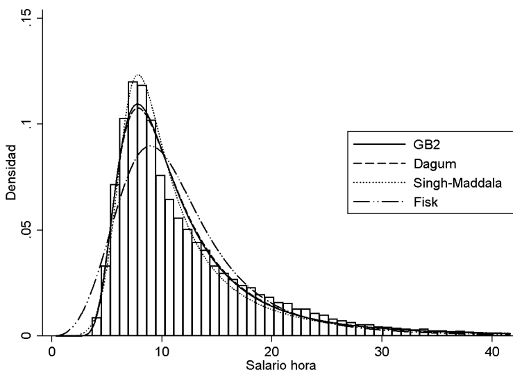
Gráfico 2: HISTOGRAMA DE LA DISTRIBUCIÓN DE LOS SALARIOS POR HORA Y FUNCIONES DE DENSIDAD DE LOS MODELOS TEÓRICOS AJUSTADOS
