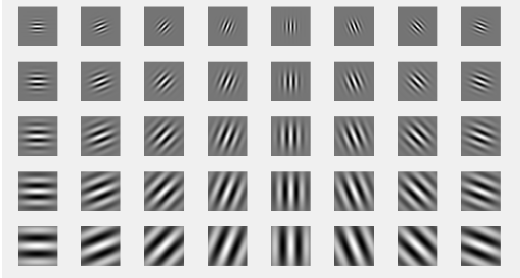
Figura 3.19: Partes reales de los 40 filtros de Gabor generados con 8 orientaciones y 5 escalas distintas
