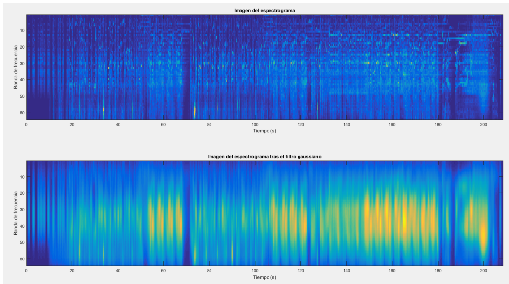
Figura 3.22: Espectrograma de Highway to Hell de AC/DC antes y después del filtrado con una máscara gaussiana de tamaño 25 y desviación típica 5
