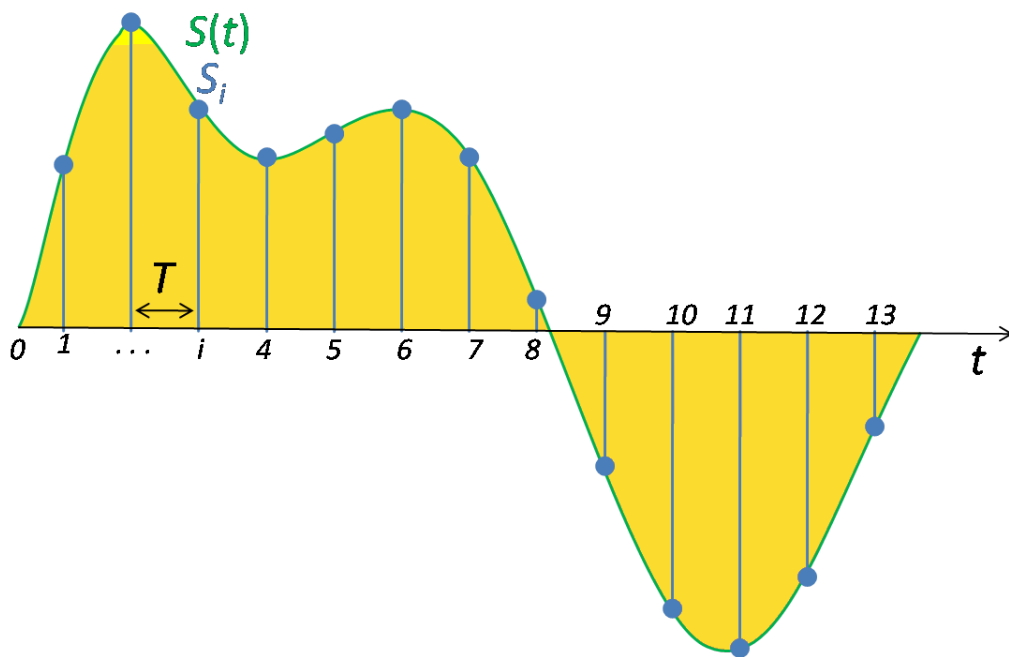
Figura 2.1: Muestreo de una señal continua para conseguir una señal digital con un período de muestreo T . La frecuencia de muestreo será f_s = \frac{1}{T}
