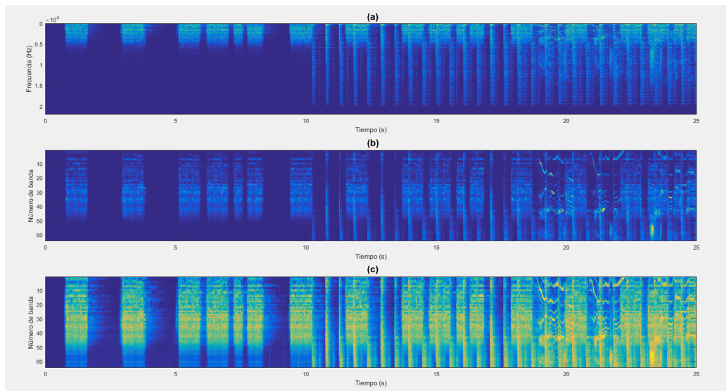
Figura 2.10: Representaciones de los primeros 25 segundos de AC/DC Highway to Hell: (a) Imagen del espectro logarítmico, (b) Imagen del espectro repartido en bandas con valores lineales, (c) Imagen del espectro repartido en bandas con valores logarítmicos. Podemos apreciar los acordes de guitarra del principio, la entrada de la batería en el segundo 10, y la voz alrededor del segundo 18
