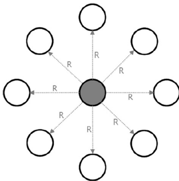
Figura 3.17: Operador LPB, representado el píxel central, sus P vecinos y la distancia R a la que están
