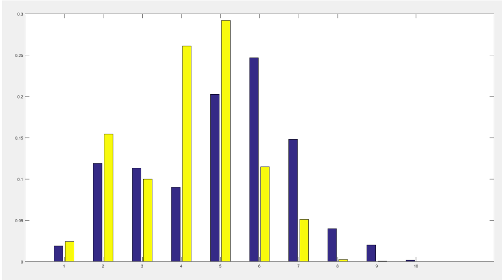
Figura 3.2: Comparación de la energía en cada subbanda para las canciones Highway to Hell de AC/DC (Azul) y Canon en Re Mayor interpretado por la Orquesta Filarmónica de Londres (Amarillo)
