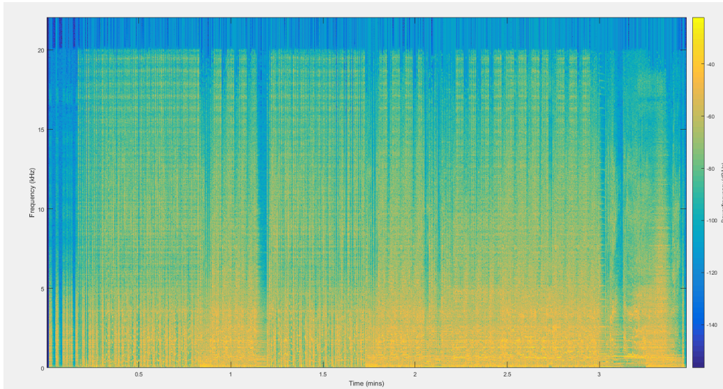
Figura 2.2: Espectrograma de la canción Highway To Hell de AC/DC. Hecho con tamaño de ventana 2048, solapamiento del 50 % y FFT de 2048 puntos
