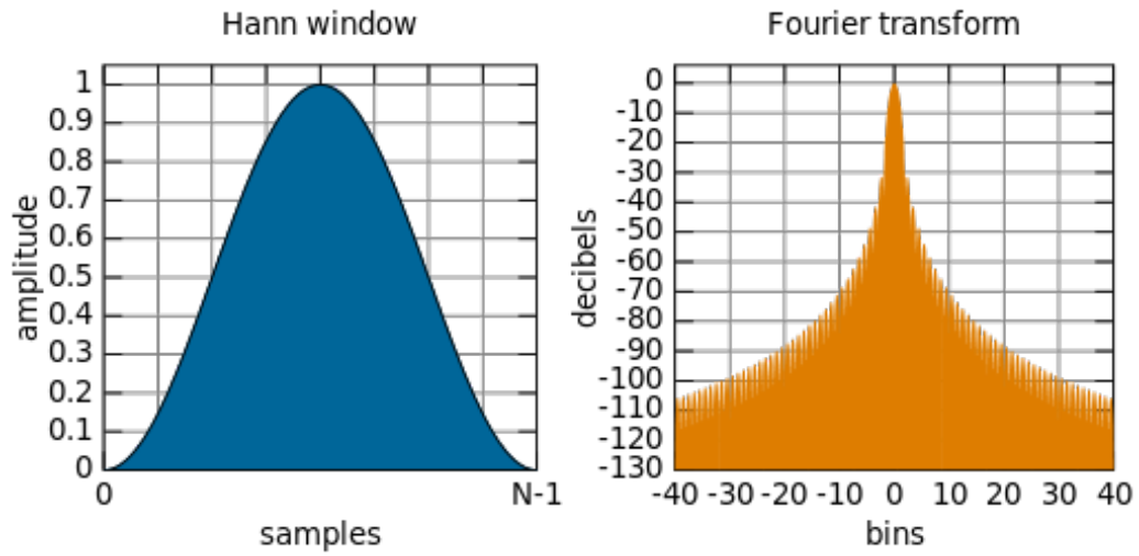
Figura 2.6: Ventana de Hann.
