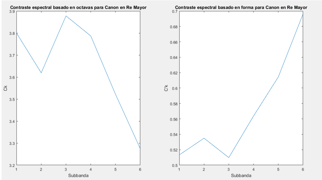
Figura 3.8: Contraste espectral de OSC y SBSC para Canon en Re Mayor interpretado por la Orquesta Filarmónica de Londres
