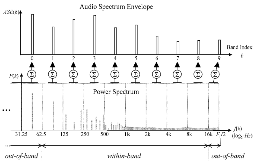
Figura 3.1: Extracción del descriptor ASE de un espectro de potencia con una resolución de una octava.
