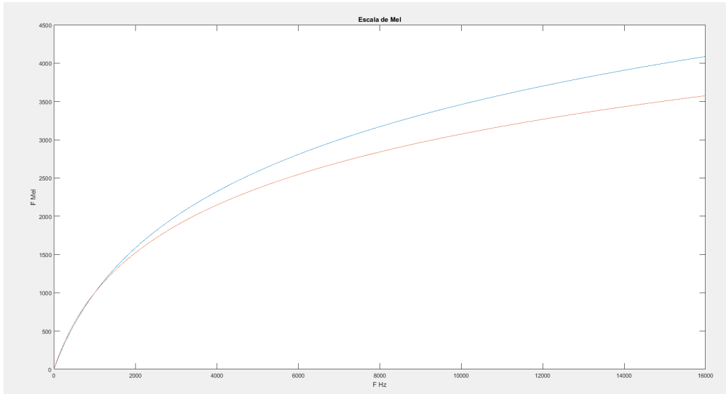
Figura 3.3: Comparación entre la frecuencia en hercios y la frecuencia de mel. En azul la fórmula de Fant y en rojo la de O'Shaugnessy
