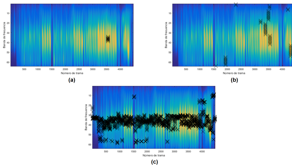
Figura 3.23: Máximos tras filtrado gaussiano de la imagen del espectrograma de Highway to Hell de AC/DC. (a) 50 máximos. (b) Máximos de cada banda. (c) Máximos de cada trama
