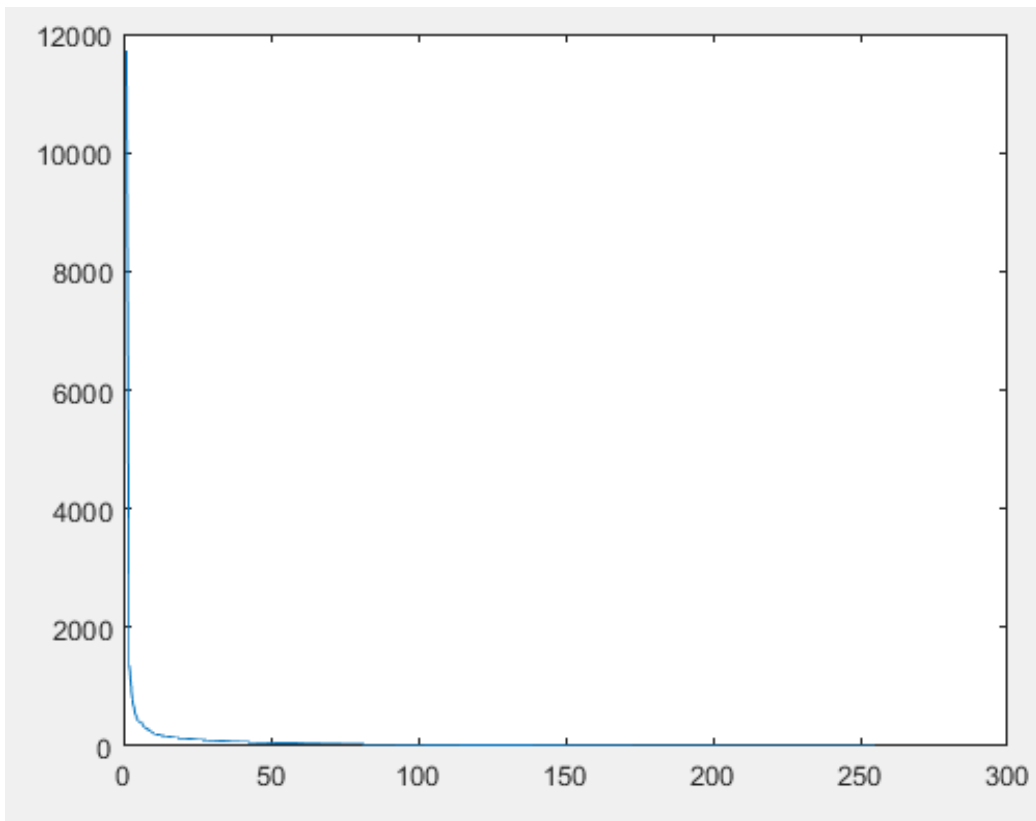
Figura 3.12: Valores singulares de la imagen 255x255 para Highway to Hell de AC/DC. Como se puede comprobar, descienden muy rápido, por eso, se puede filtrar muy fuertemente sin perder la información principal
