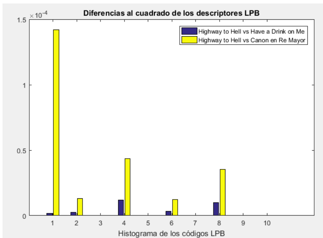
Figura 3.18: Comparación de las diferencias al cuadrado de los 10 primeros códigos de los descriptores LPB entre Highway to Hell y Have a Drink on Me, dos canciones de AC/DC y entre Highway to Hell y Canon en Re Mayor
