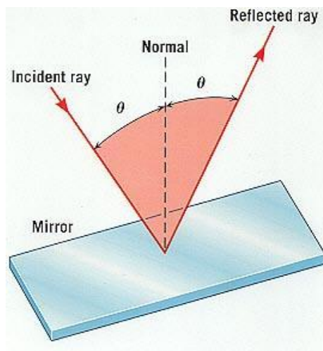
Figura 2: Reflexión de un rayo de luz.
