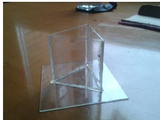
Figura 13: Prisma obtenido en el laboratorio
