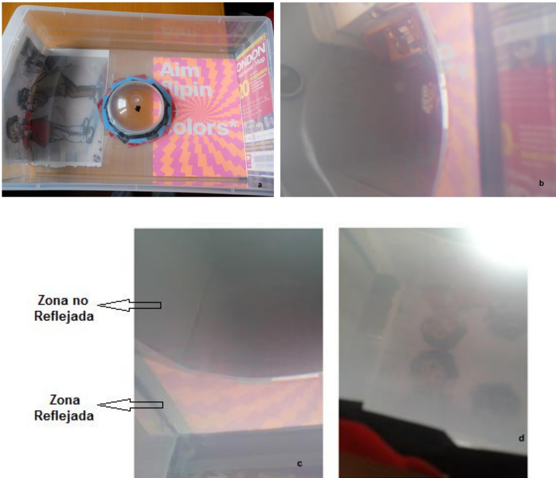
Figura 10: Experimento de reflexión total
