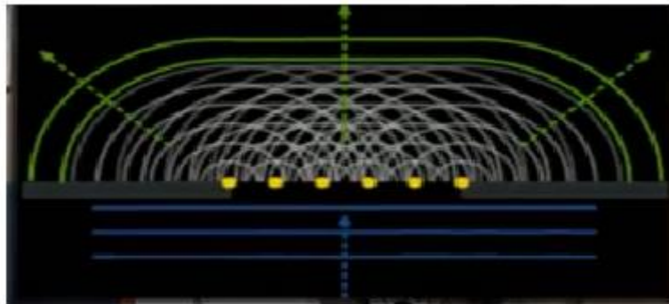
Figura 18: Fenómeno de difracción
