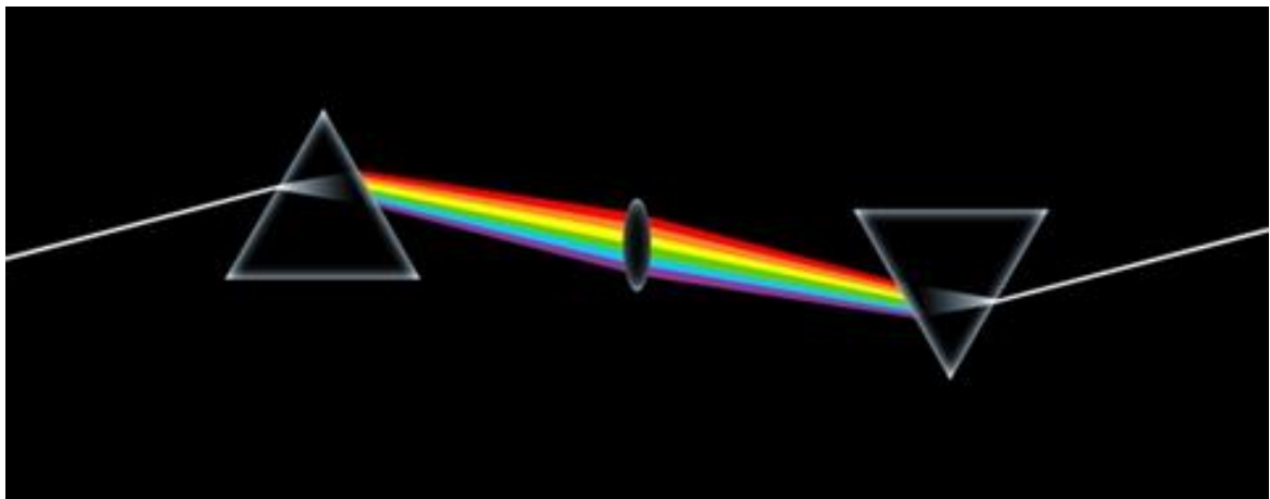
Figura 11: Descomposición y composición de la luz
