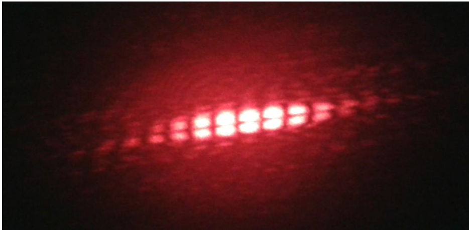
Figura 17: Resultado de la interferencia de luz láser sobre una doble rendija.
