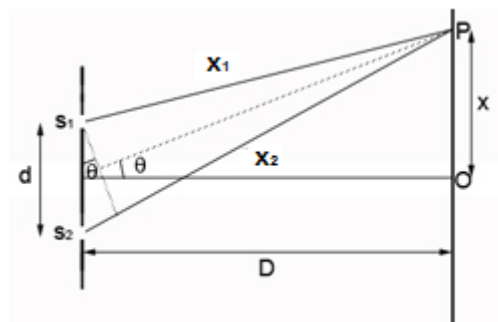
Figura 15: Interferencia de las ondas $X_1$ y $X_2$ en el punto P
