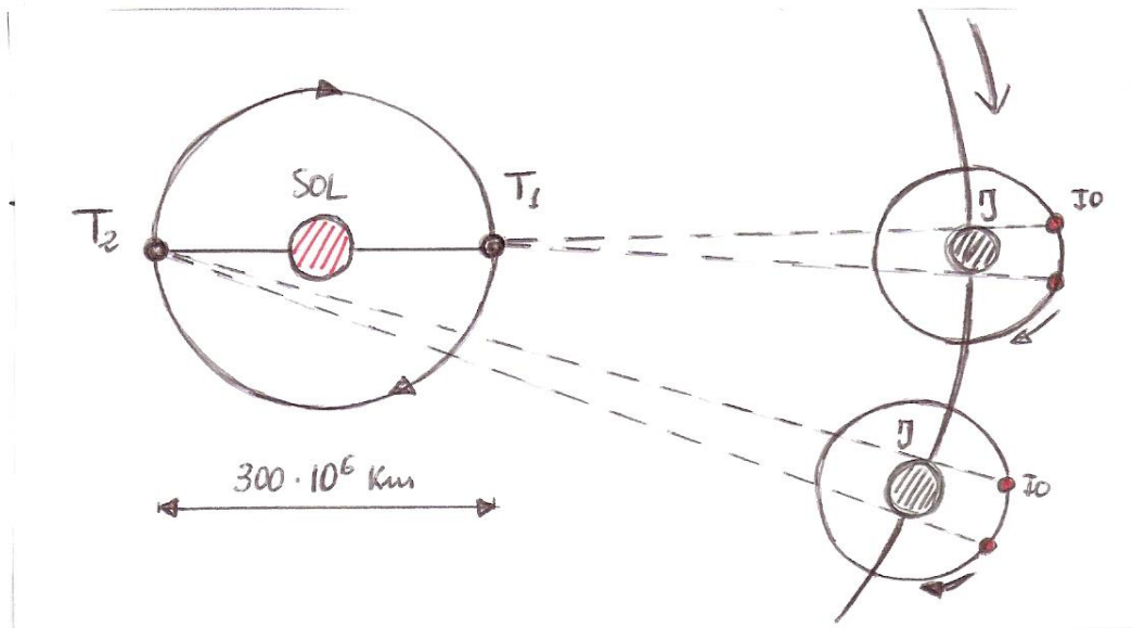
Figura 1: Fundamento del experimento de O.Romer.
