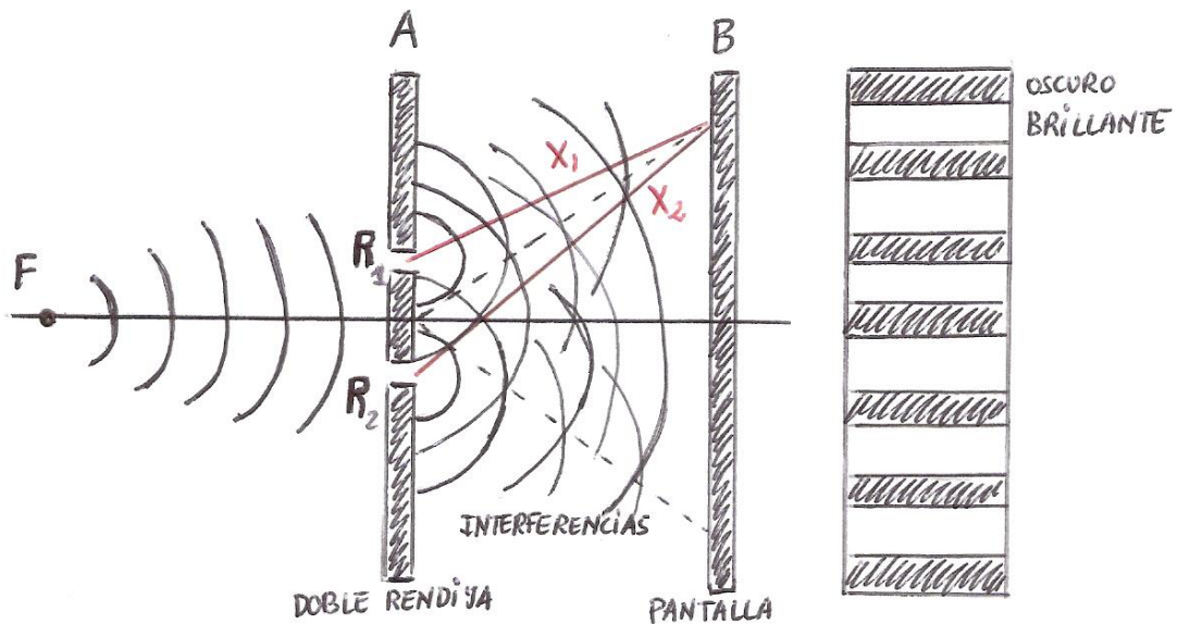
Figura 14: Experimento de la doble rendija
