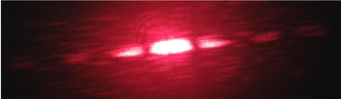
Figura 19: Interferencia a través de una rendija.
