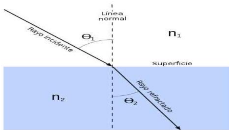
Figura 4: Refracción de la luz.
