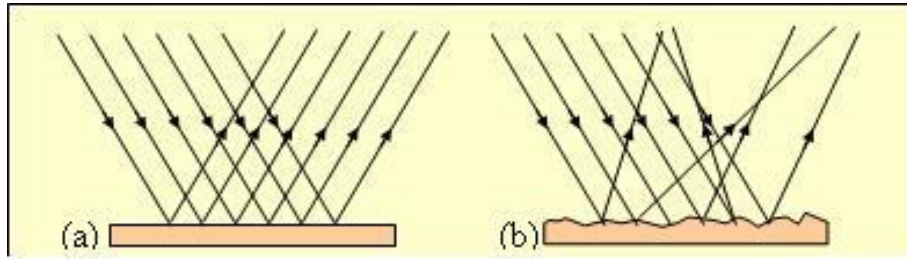
Figura 3: Reflexión dirigida (a) y difusa (b)
