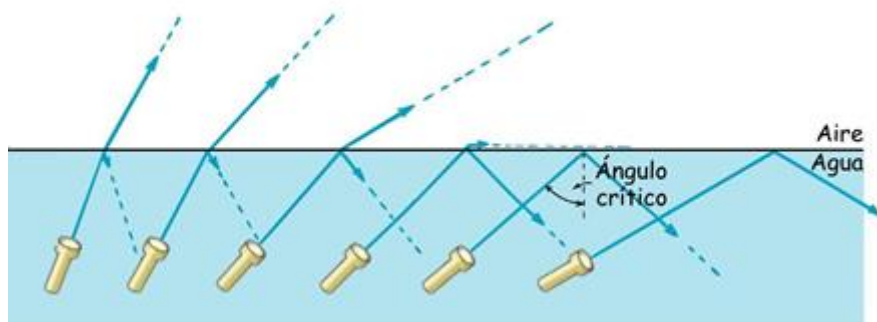
Figura 5: Ilustración del ángulo límite
