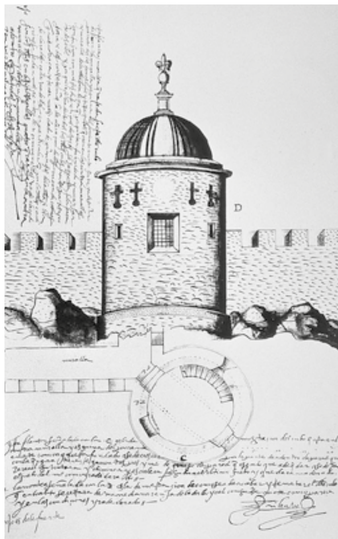
FIG. 159 Proyecto de reformas en el castillo de Piedrabuena, según condiciones y trazas formadas por Juan Bravo, en 1593. Madrid, Archivo Histórico Nacional, Órdenes Militares, Consejo de Órdenes, Archivo de Toledo [pleito núm. 28.793m s/f]
