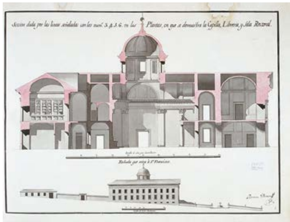
FIG. 62 Colegio Imperial de Alcántara en Salamanca. Proyecto del Colegio de la Orden de Alcántara de Salamanca presentado por don Ramón Durán, 1791. Archivo Histórico Nacional. Órdenes Militares, Mapas y Planos, n.º 22 (antes leg. 3677º, n.º 11). 2. Plano de la planta baja del proyecto
