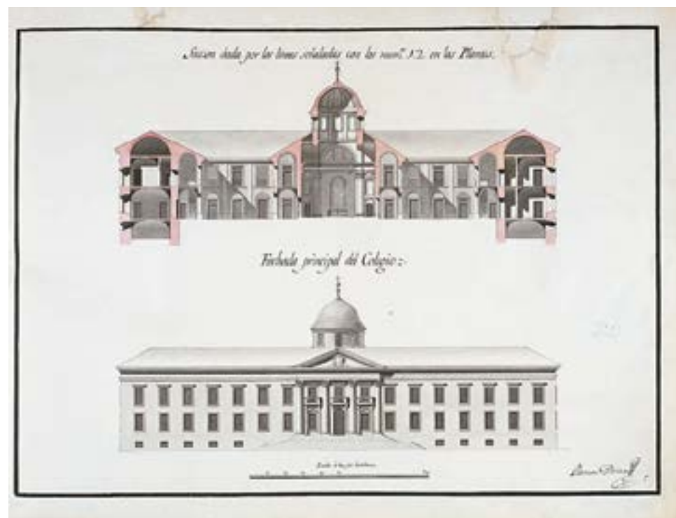
FIG. 63 Colegio Imperial de Alcántara en Salamanca. Proyecto del Colegio de la Orden de Alcántara de Salamanca presentado por don Ramón Durán, 1791. Archivo Histórico Nacional. Órdenes Militares, Mapas y Planos, n.º 22 (antes leg. 3677º, n.º 11). 5. Sección transversal del edificio; y fachada principal del Colegio
